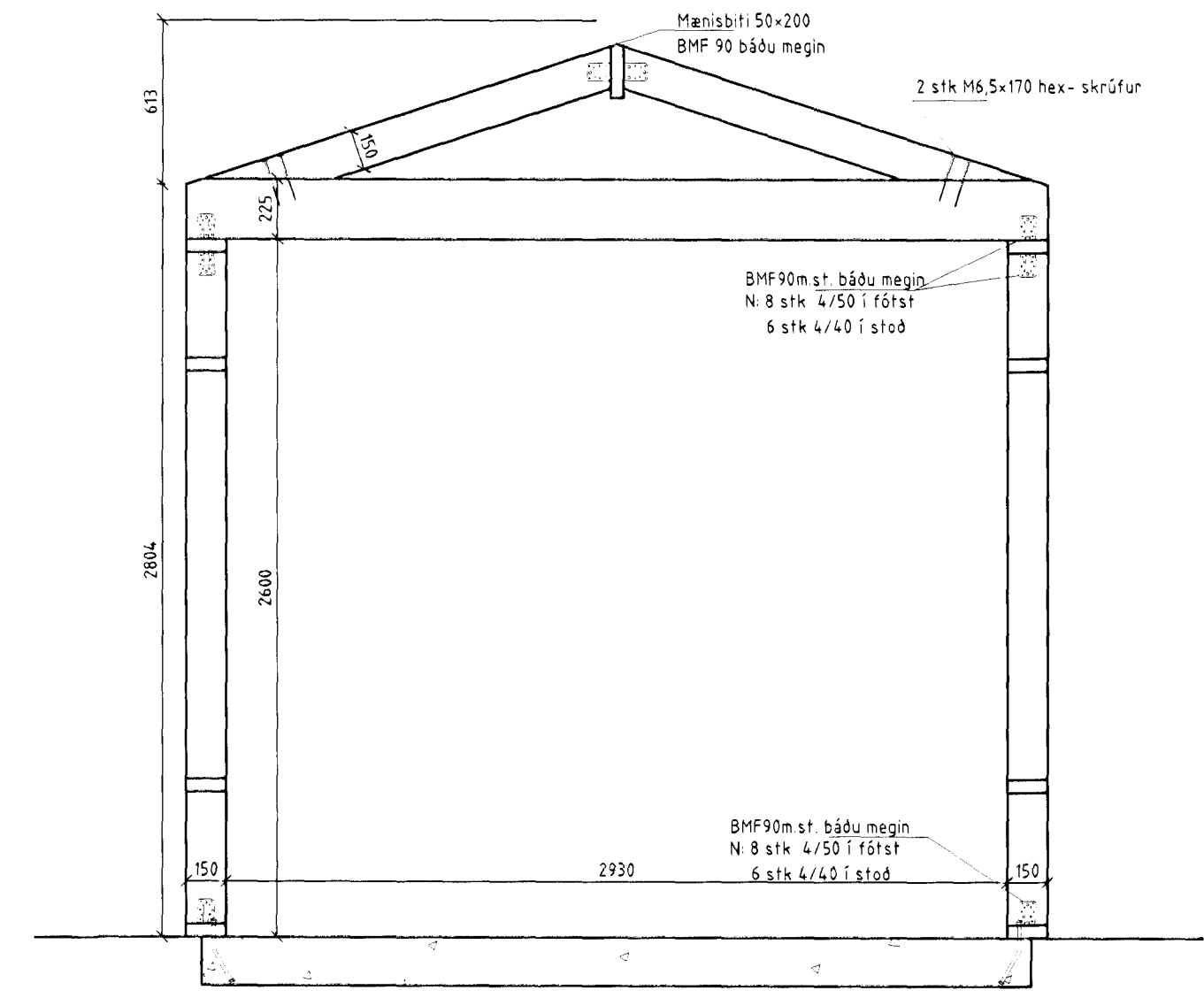
DVERSNIÐ E, 1-25
