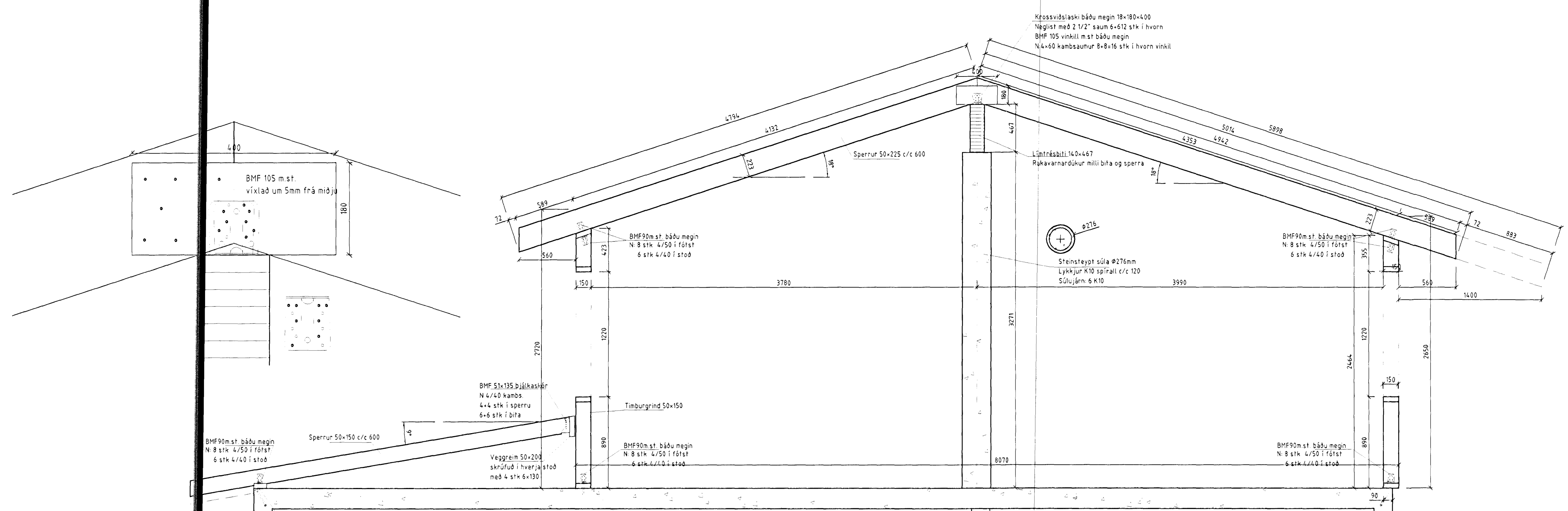
DVERSNIÐ A, 1:25
