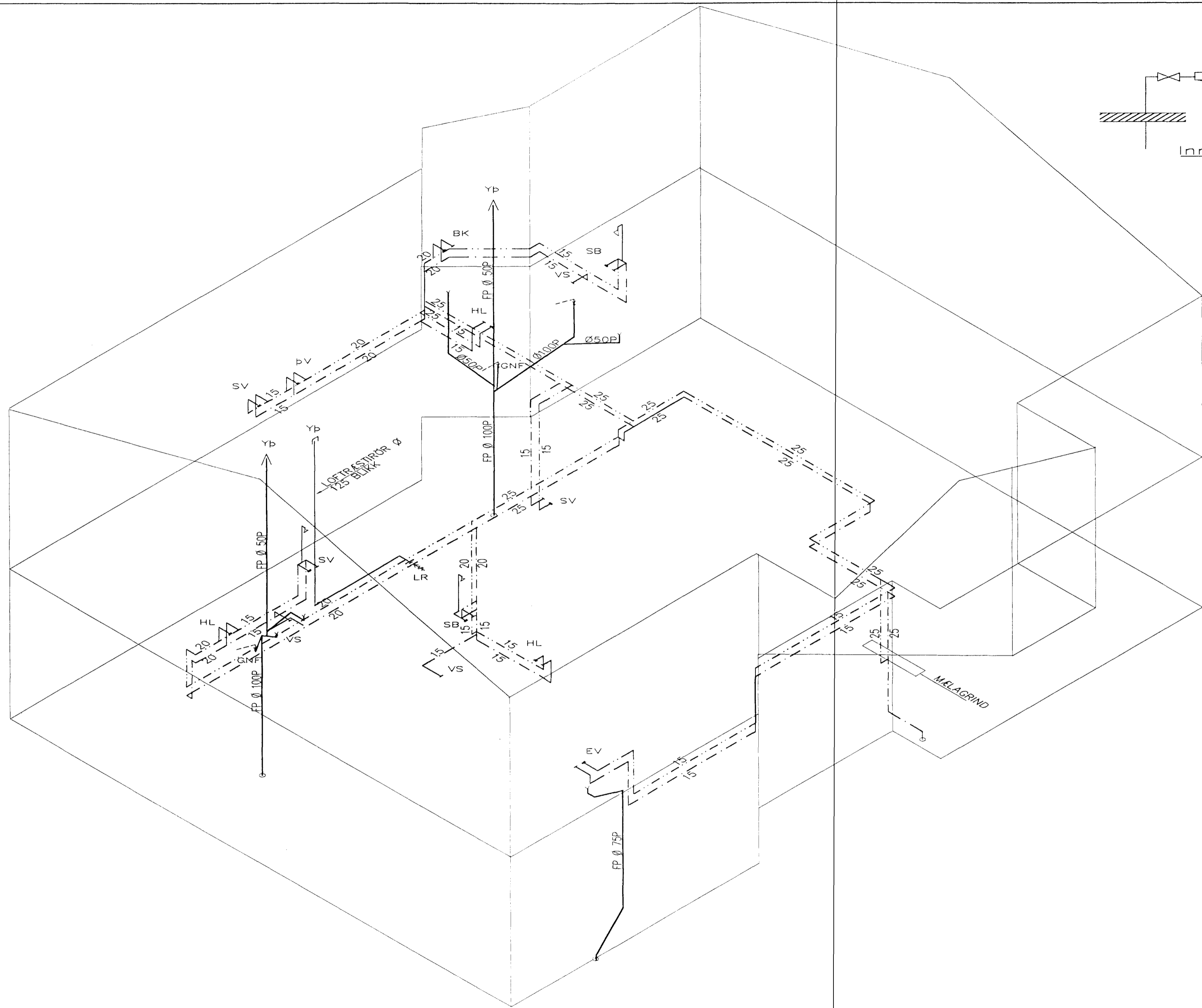
RÚMMYND VATNS OG FRÁRENNISLAGNA 1:50
