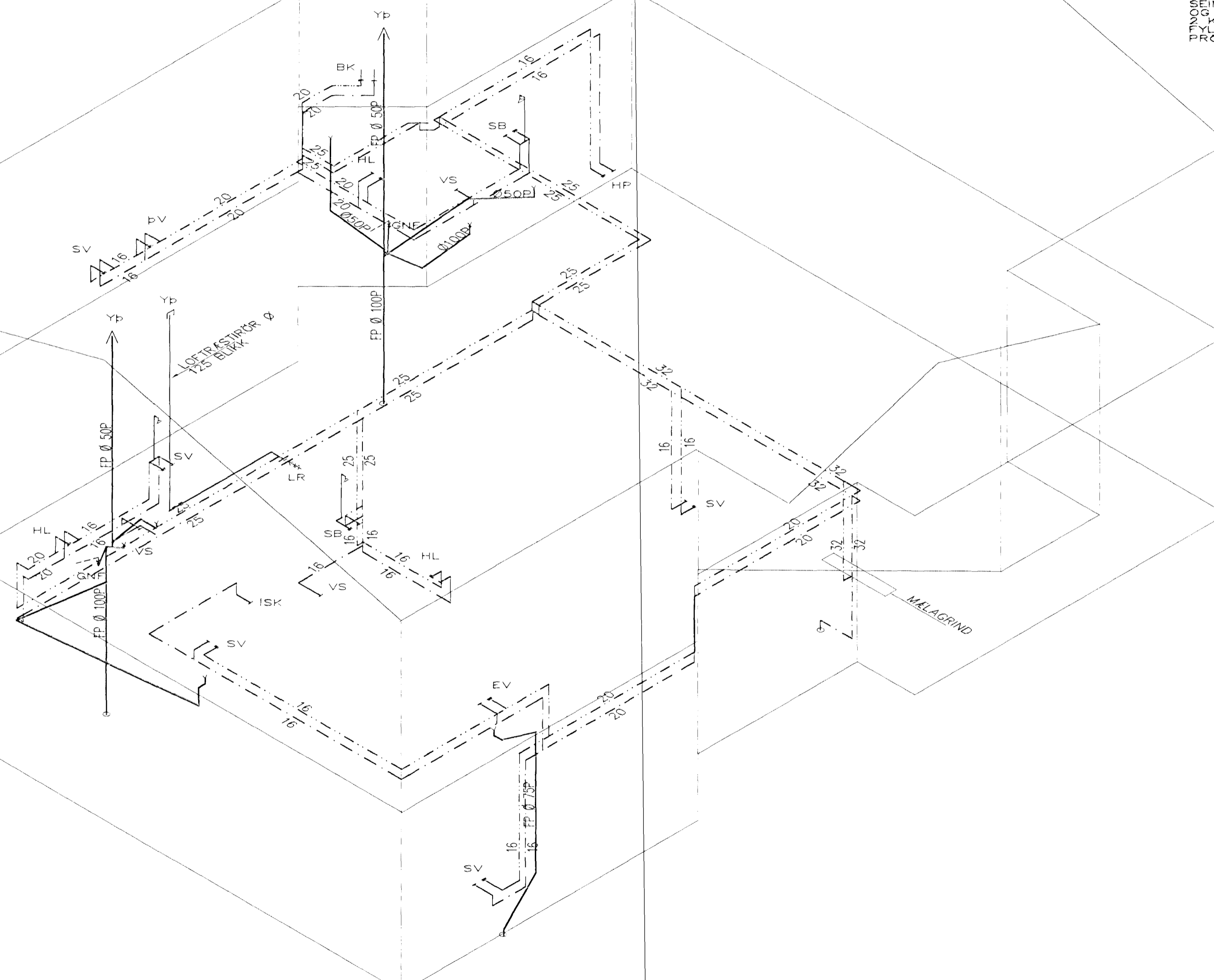
RÚMMYND VATNS OG FRÁRENNSLISLAGNA 1:50
