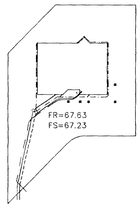
AFSTÖÐUMYND 1:500
