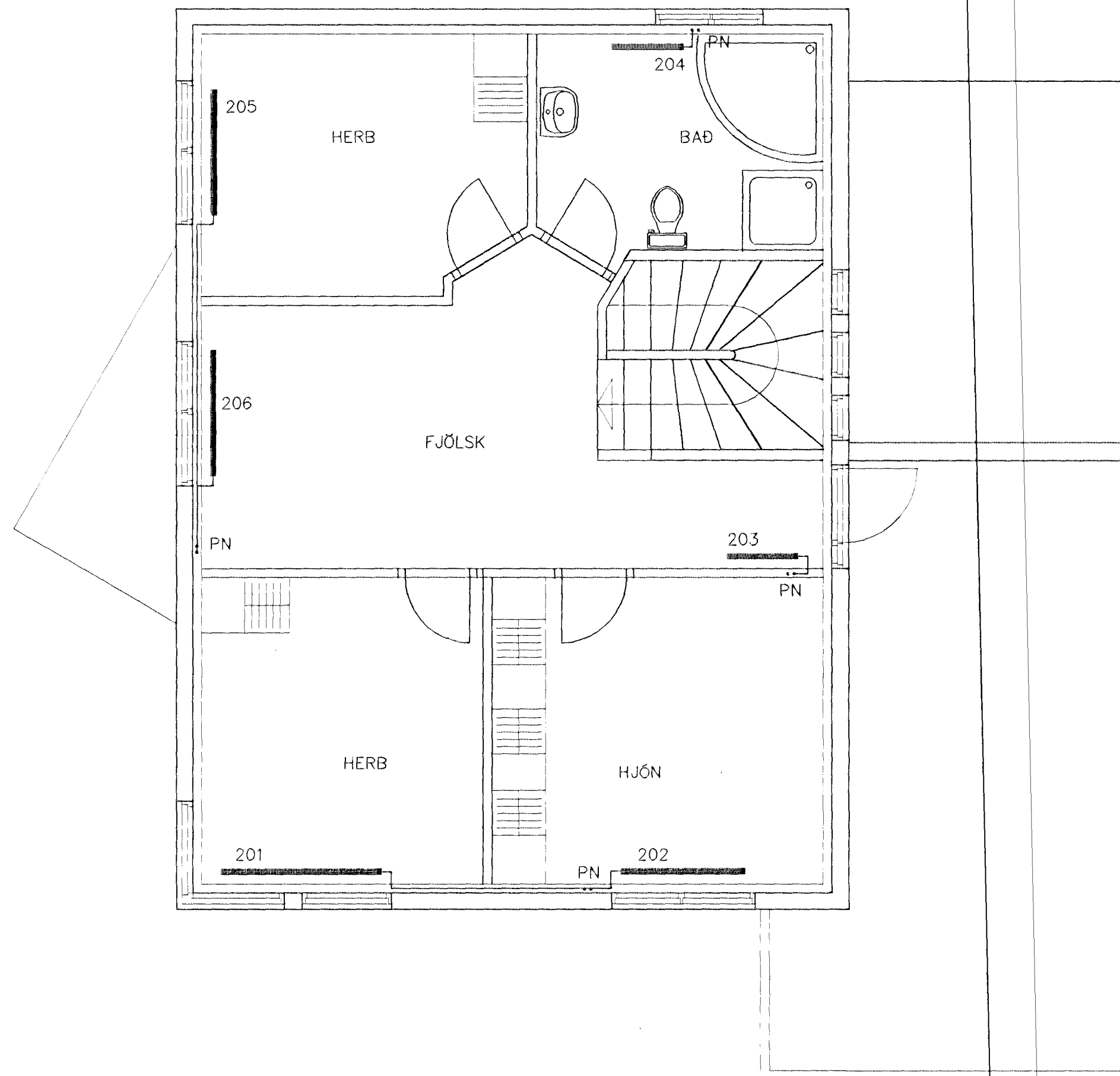
GRUNNMYND 2 HÆÐAR 1:50
