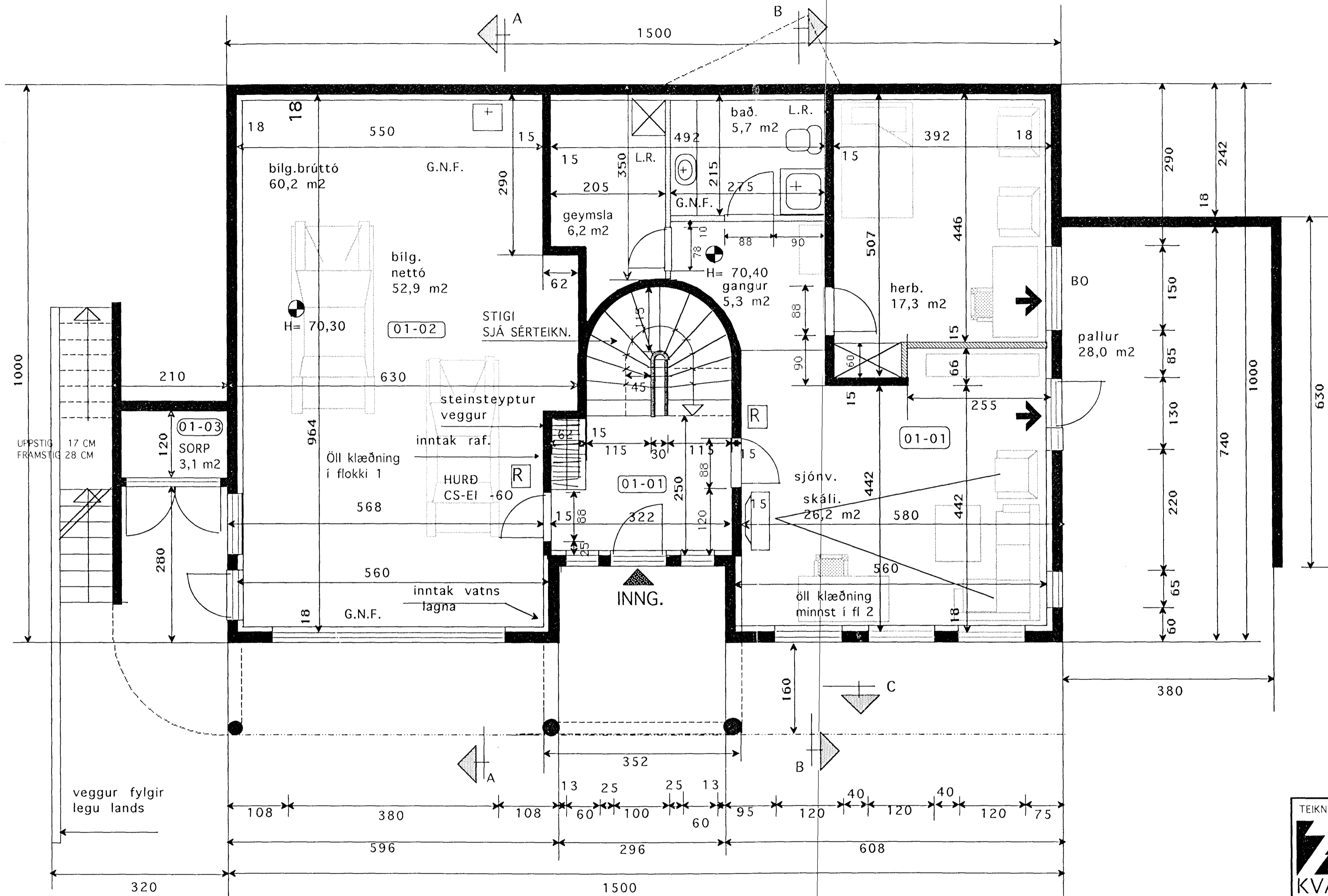
GRUNNMYND 1 HÆÐ
