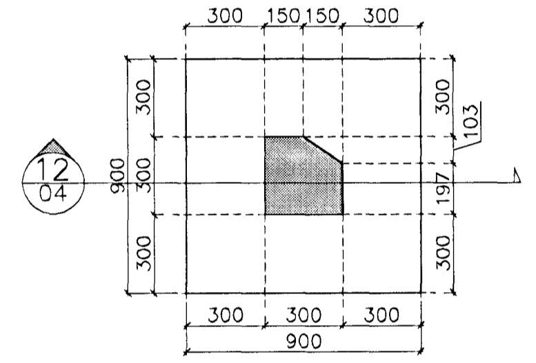
A-01 Deili, 1:20
