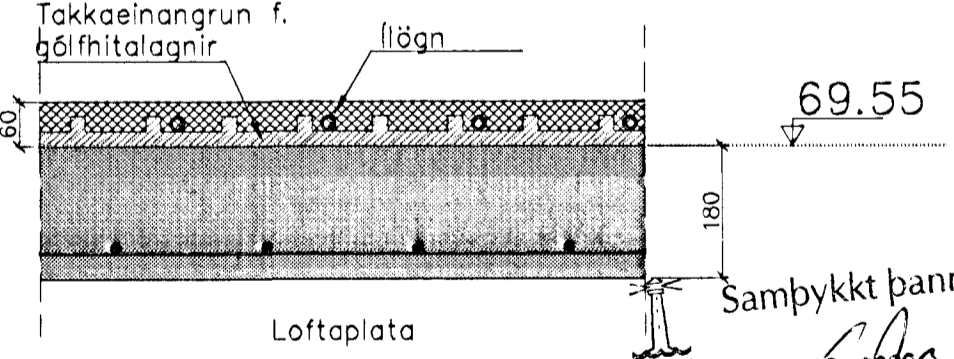
Snið í gólfhitalögn á efrihæð Mkv. 1:10
