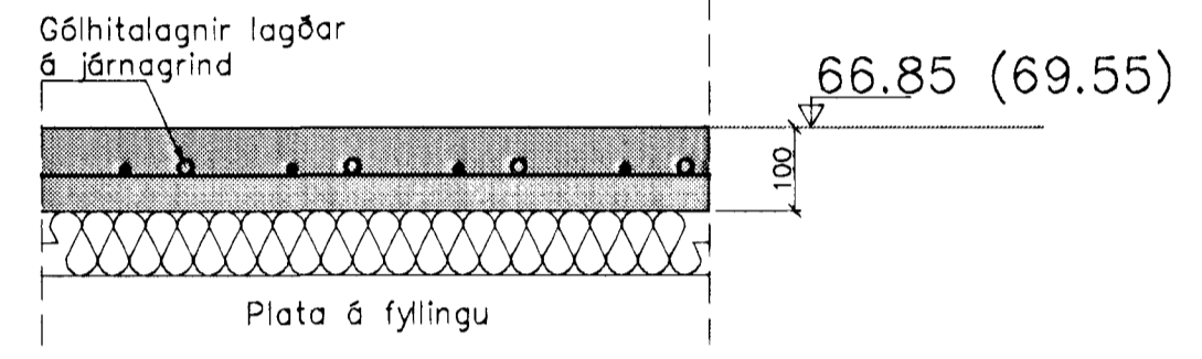
Snið í gólfhitalögn á jarðhæð og í bílskúr Mkv. 1:10
