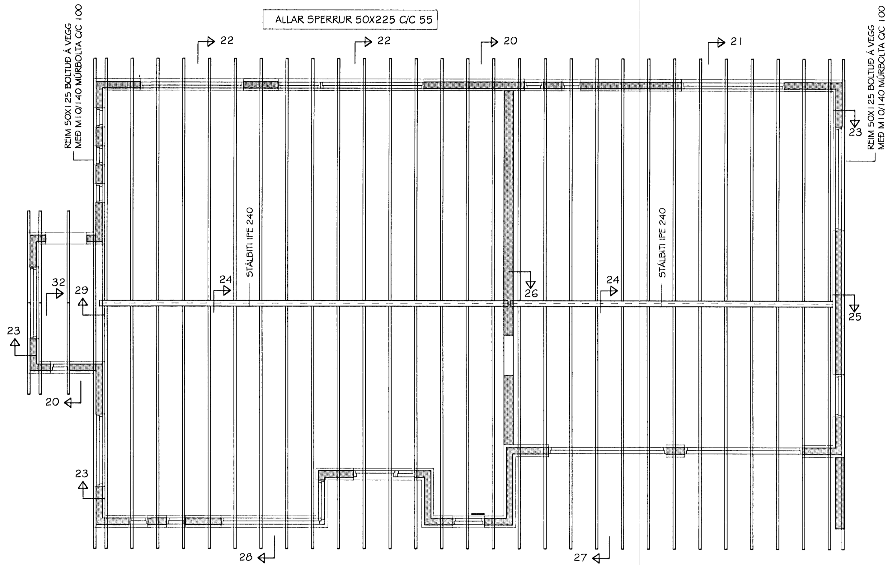
GRUNNMYND ÞAKVIÐA MKV. 1:50
