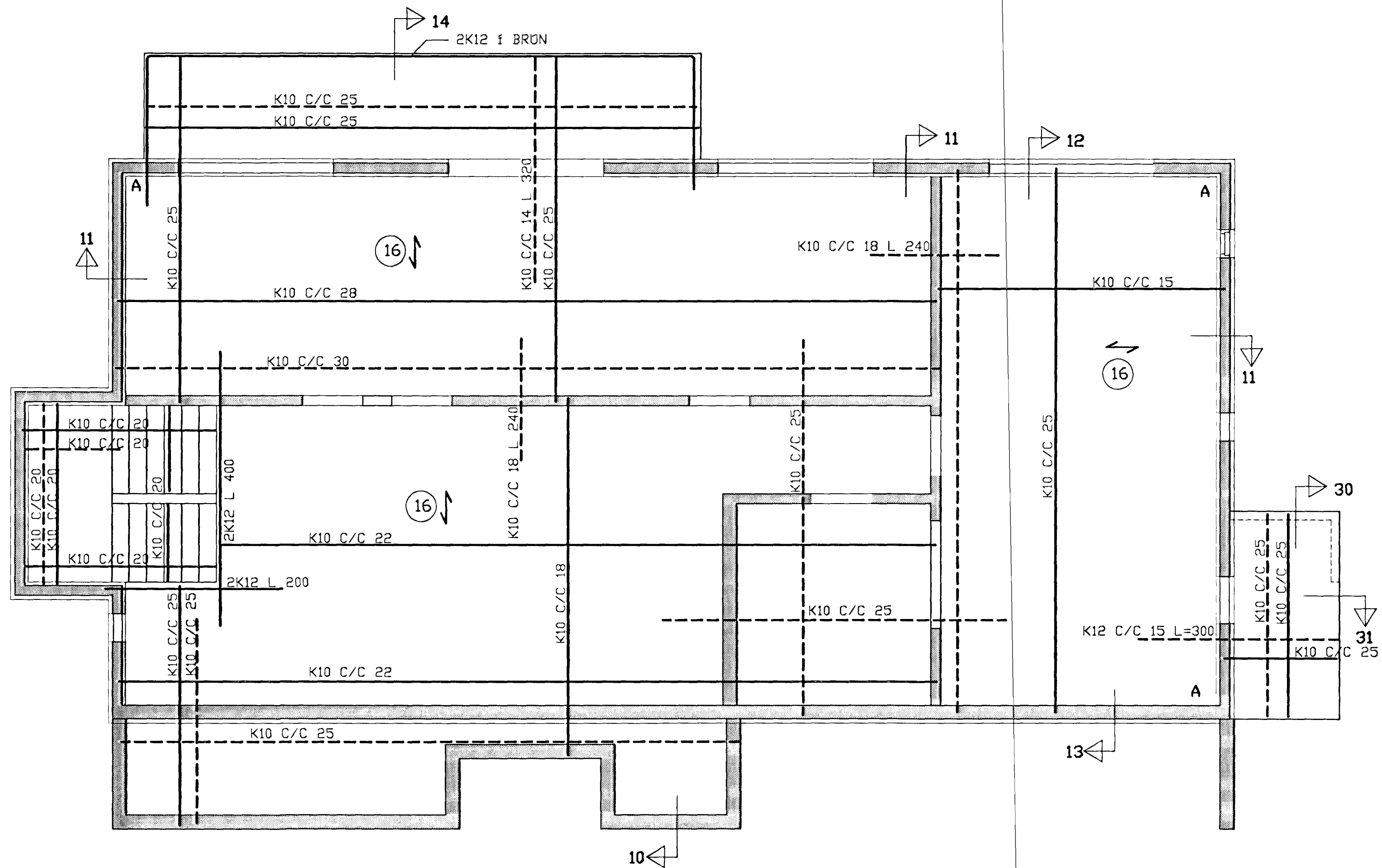
JÄRN Í PLÖTU YFIR NEDRI HÆÐ MKV. 1:50
