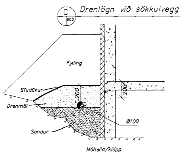
Frágangur á dreni (þerrilögn) við sökkulvegg
