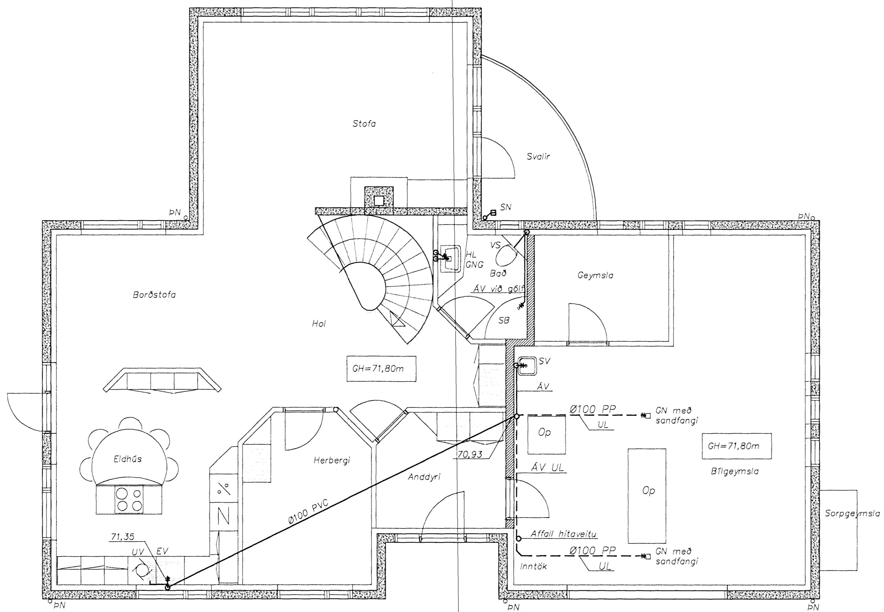
Grunnmynd, aðalhæð Málkvæði 1:50
