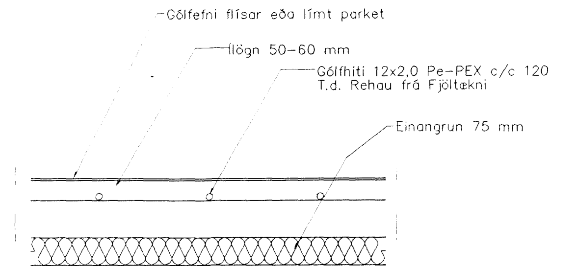
GÓLFHITALAGNIR SNIÐ 1:20
