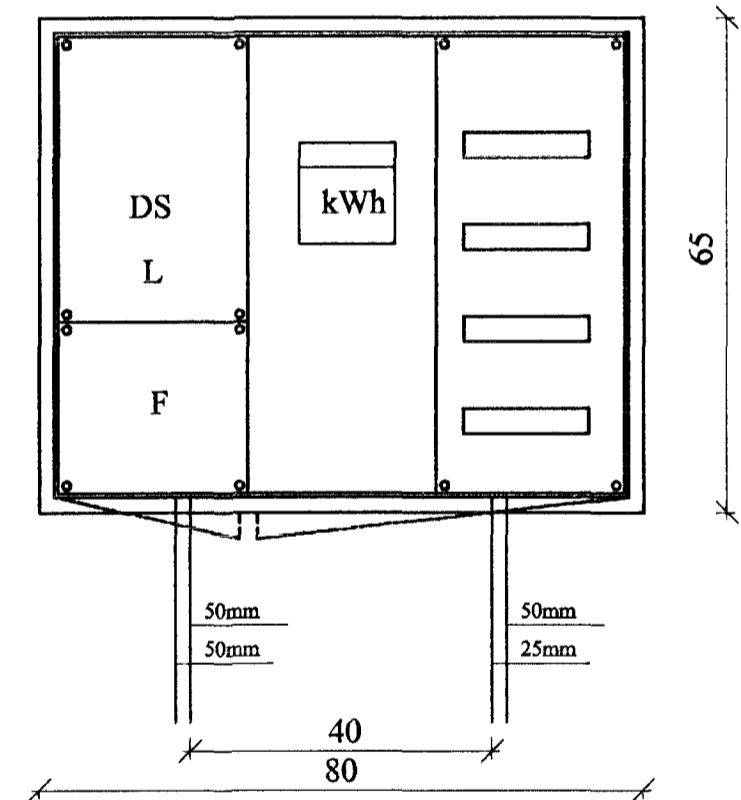
'Utlit töflukassa TA mkv. 1:10
