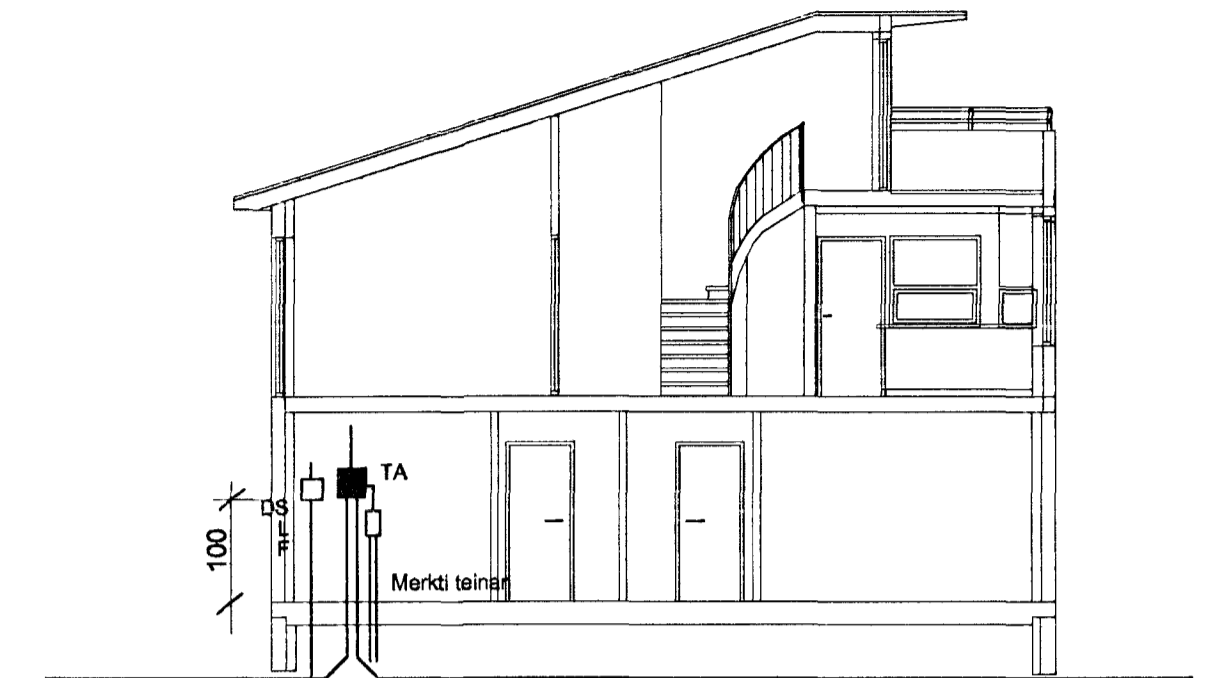
Snið a-a mkv. 1:100
