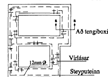
Grunnmynd sökkulveggja
