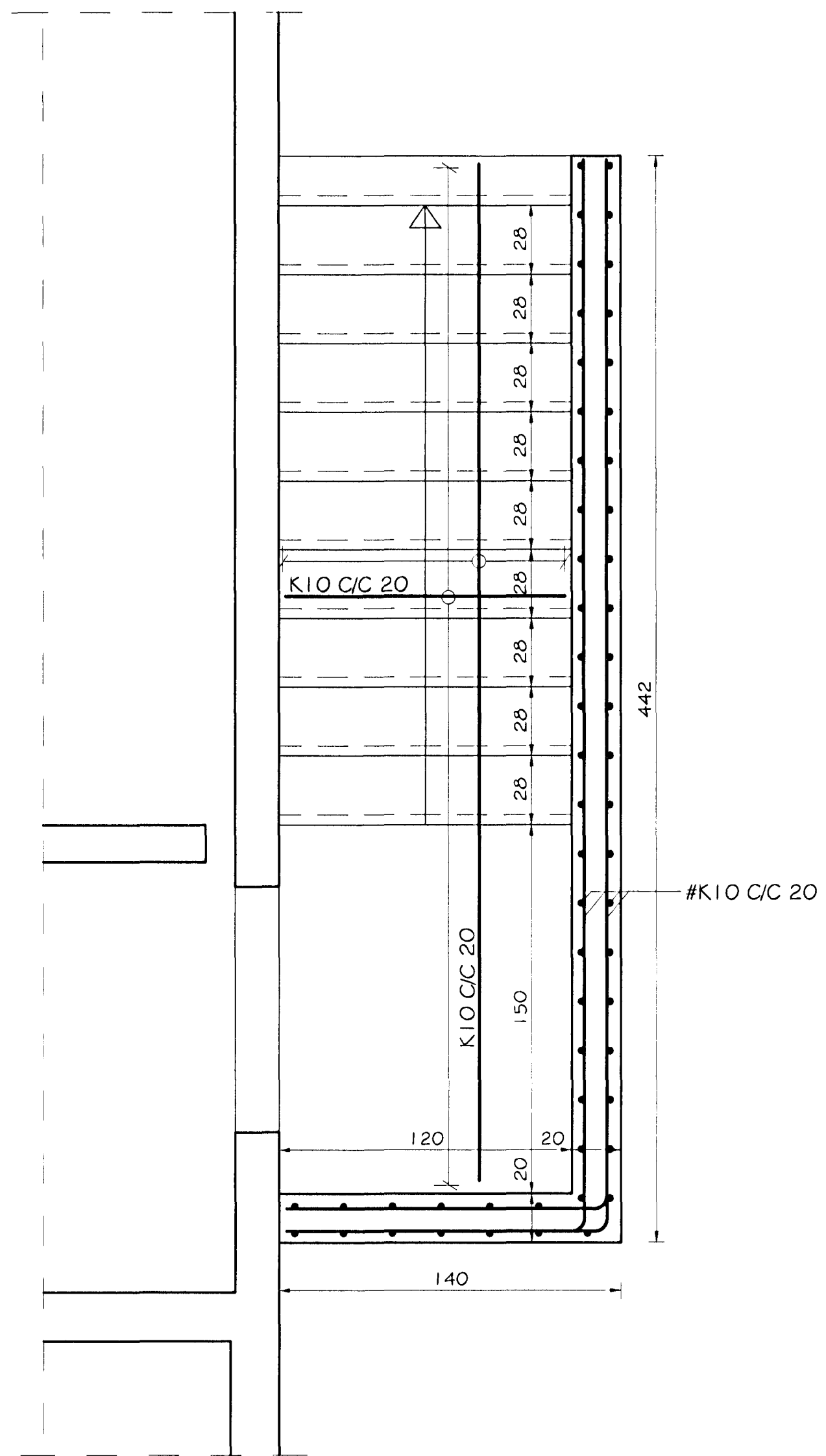
STIGI ÚT ÚR NEDRI HÆÐ - GRUNNMYND MKV. 1:20
