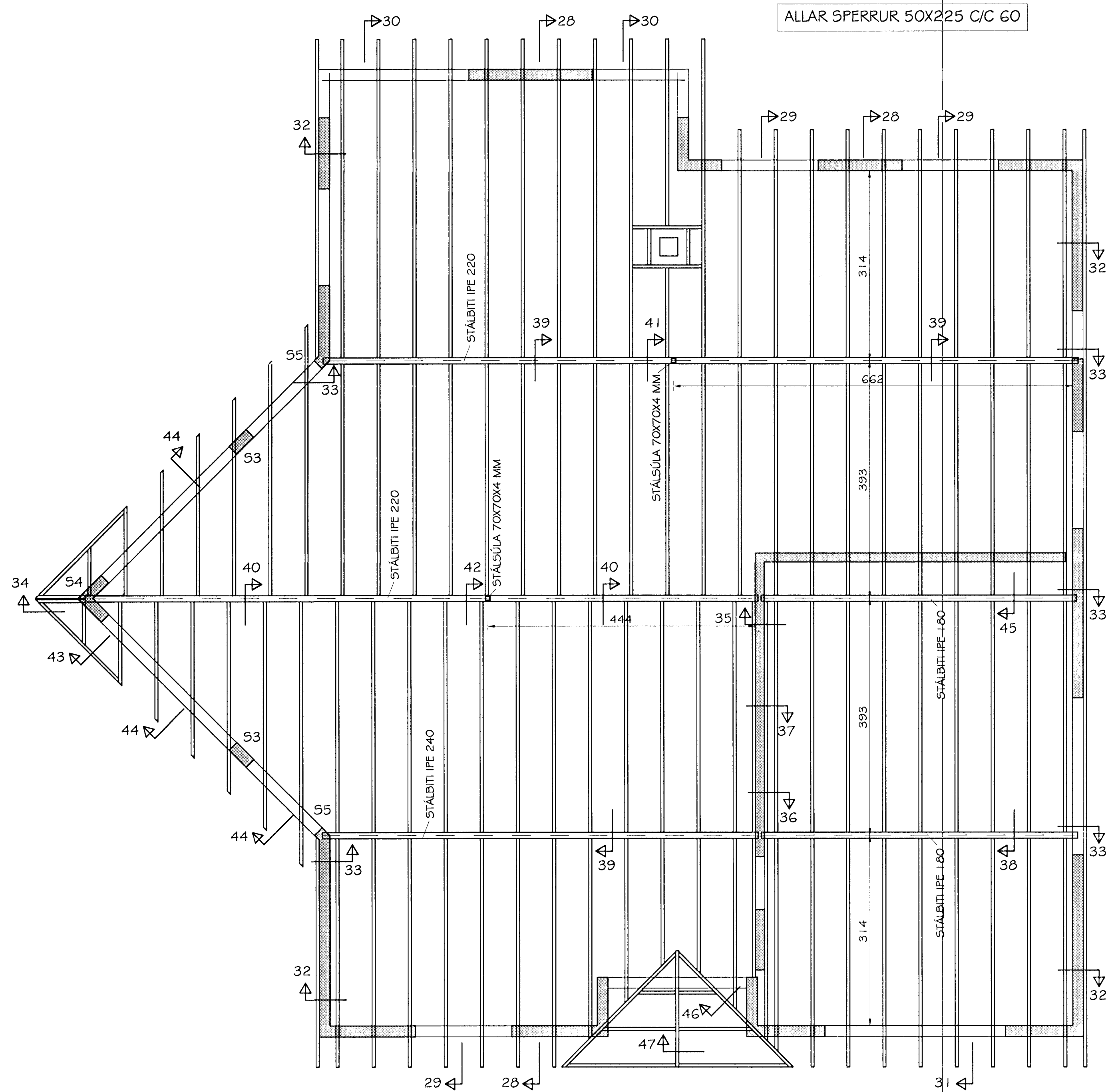
GRUNNMYND PAKVIDA MKV. 1:50
