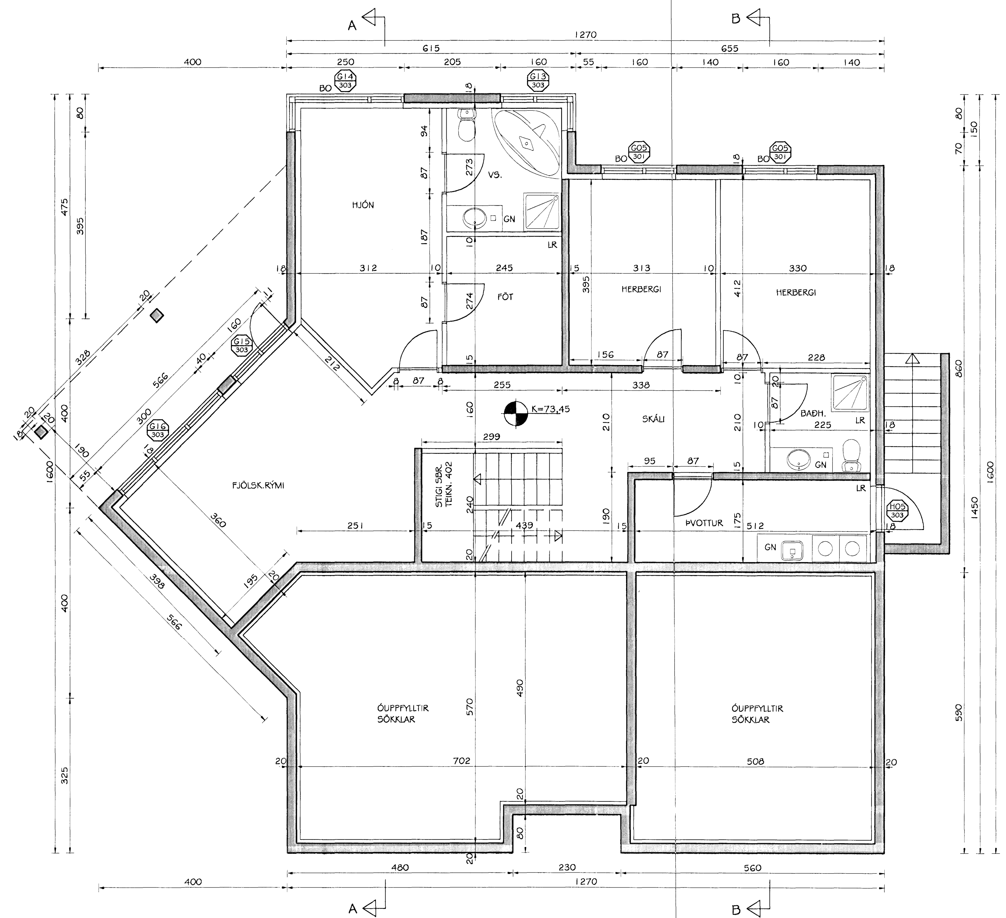
GRUNNMYND NEDRI HÆÐAR MKV. 1:50
