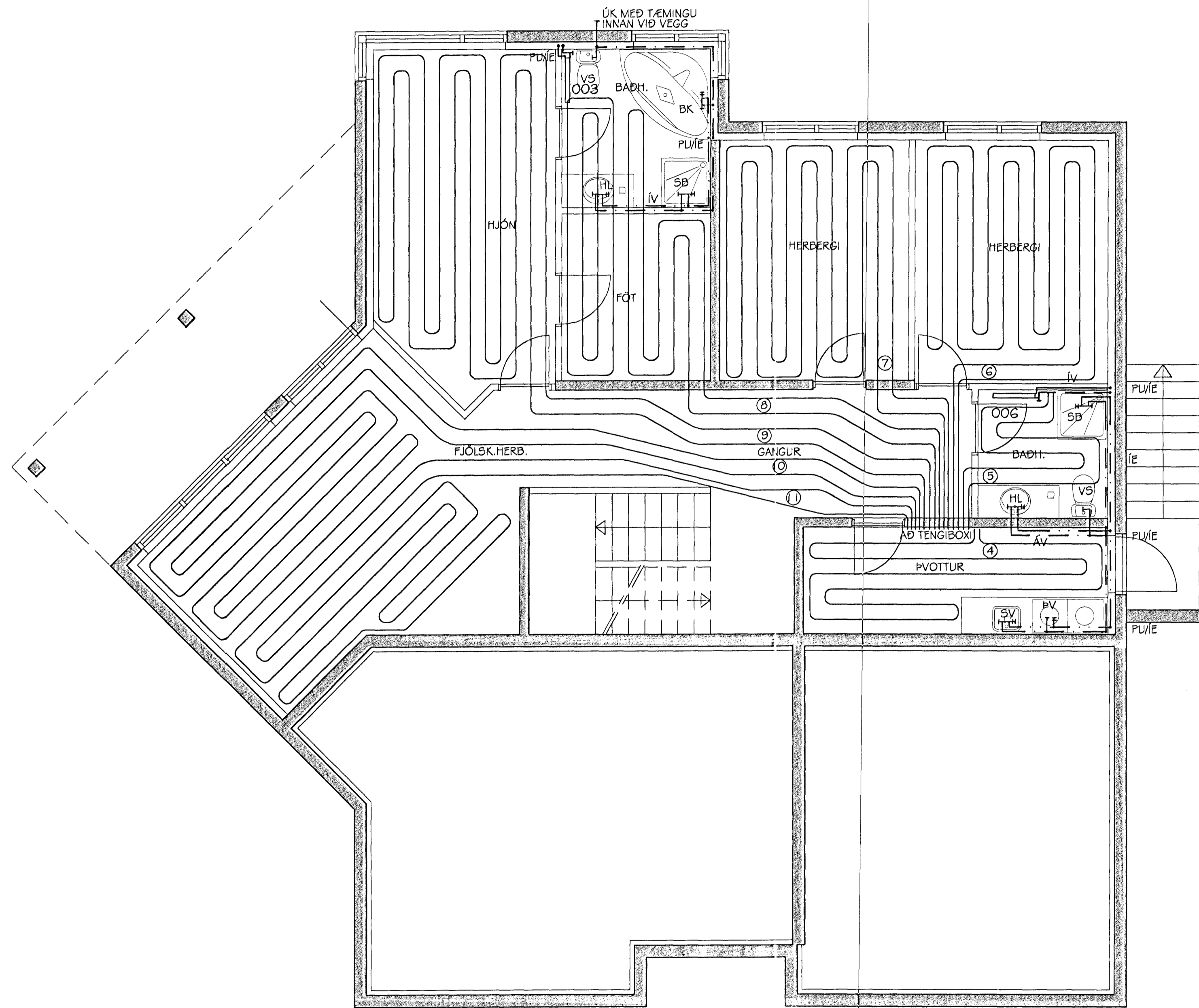
NEYSLUVATNS- OG HITLAGNIR GRUNNMYND NEDRI HÆÐAR MKV. 1:50
