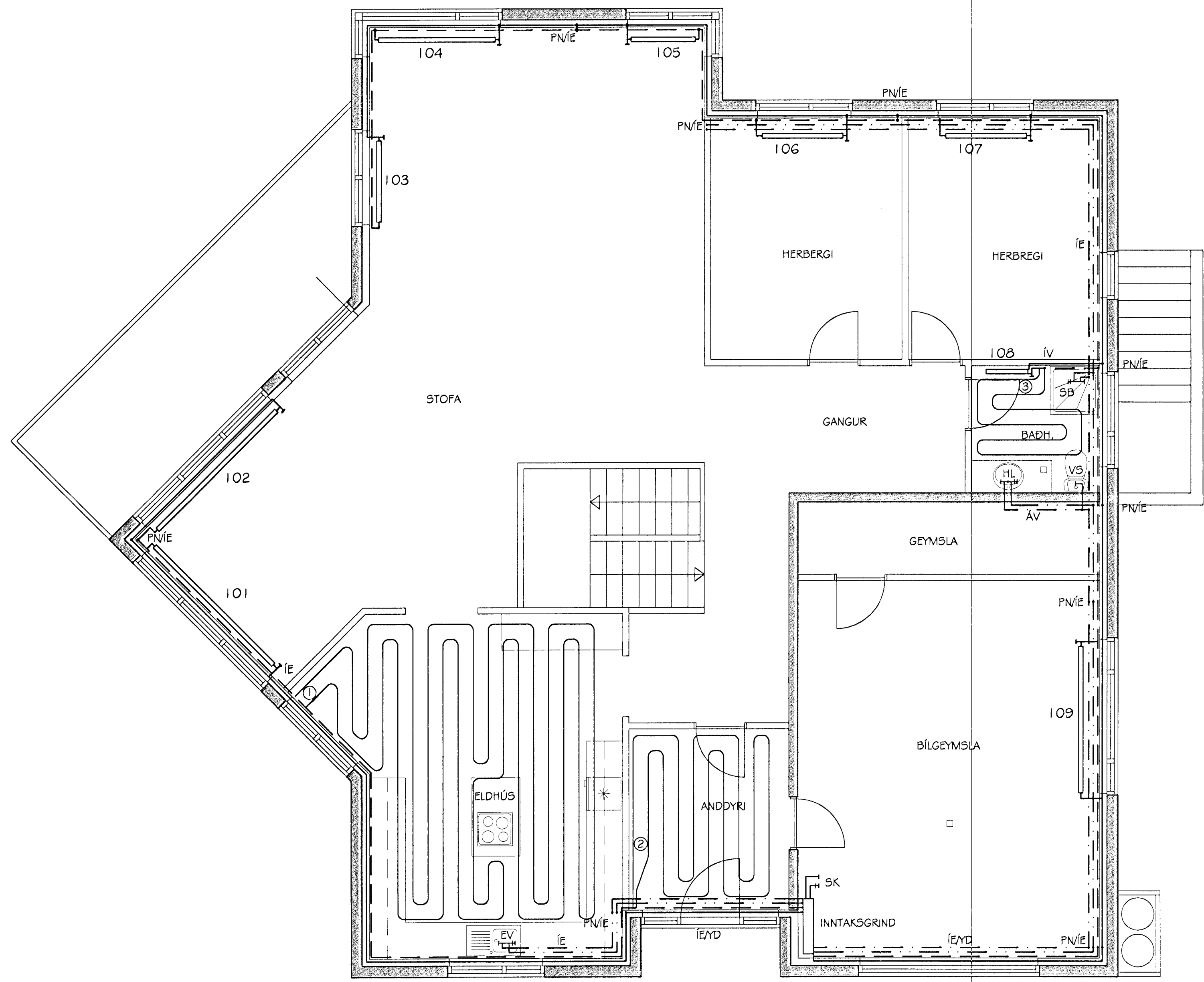
NEYSLUVATNS- OG HITALAGNIR GRUNNMYND EFRI HÆÐAR MKV. 1:50
