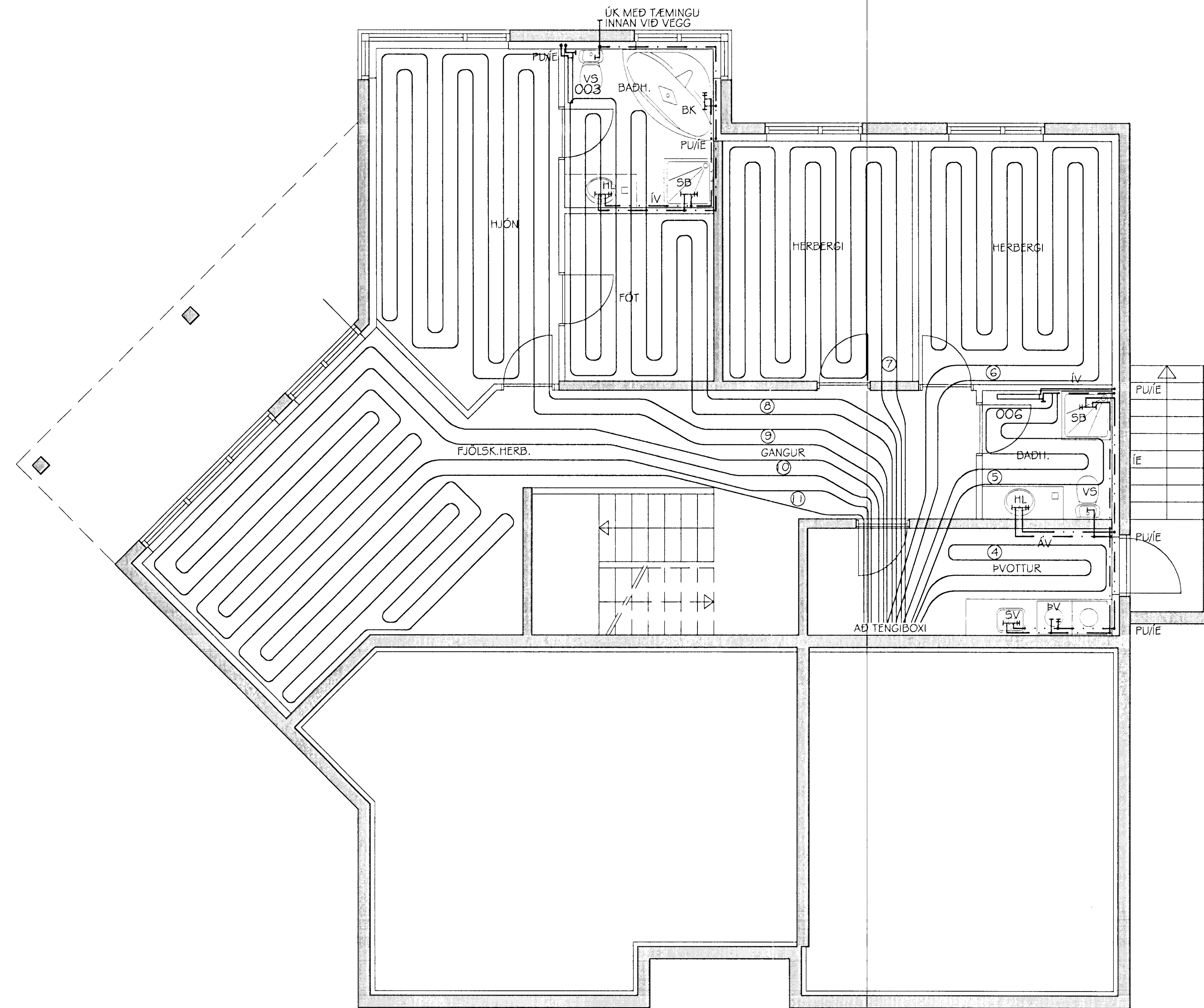
NEYSLUVATNS- OG HITALAGNIR GRUNNMYND NEDRI HÆÐAR MKV. 1:50
