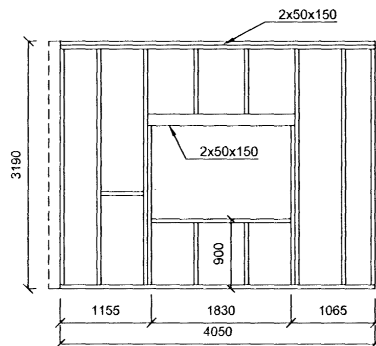
GRIND NR. 25 MKV. 1:50
