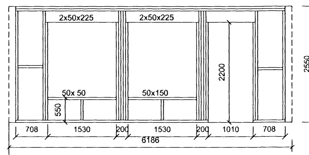
GRIND NR. 5 MKV. 1:50
