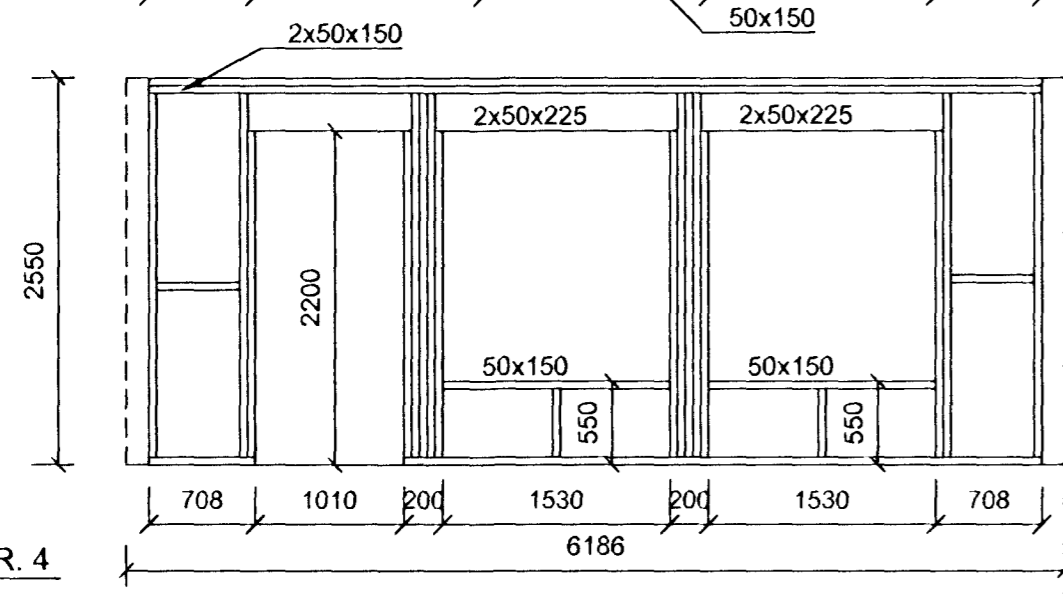
SNID MKV. 1:20
