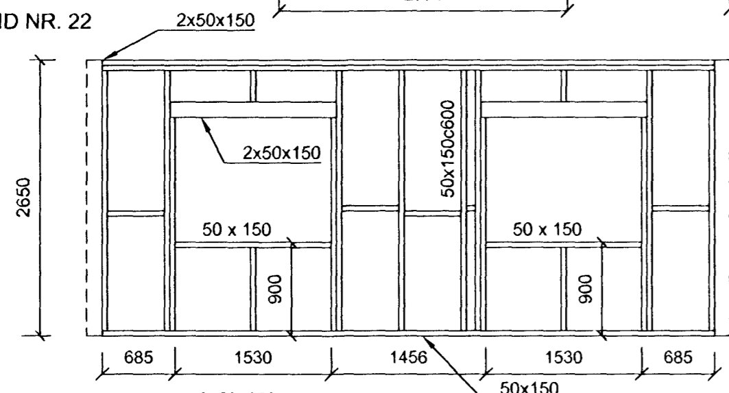
GRIND NR. 22 MKV. 1:50
