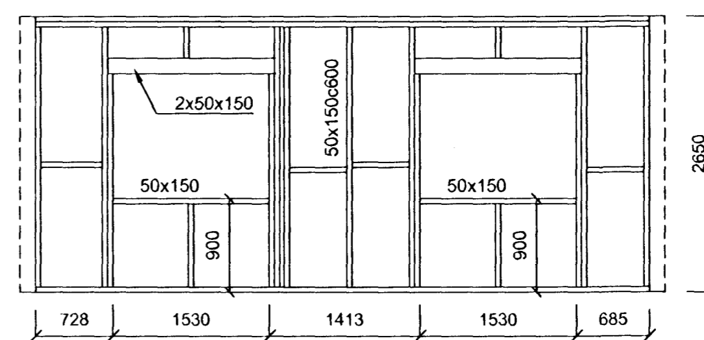
GRIND NR. 27 MKV. 1:50
