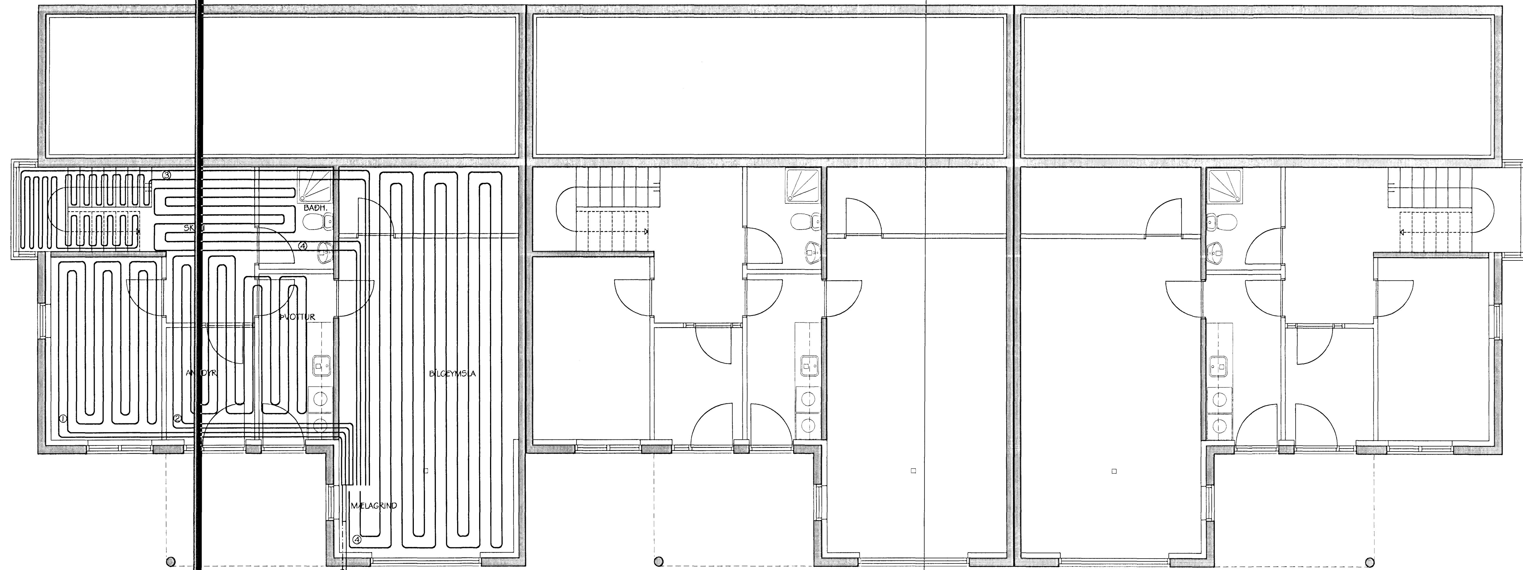
GAUKSÁS 7 HITALAGNIR GRUNNMÝND NEÐRI HÆÐA MKV. 1:50
