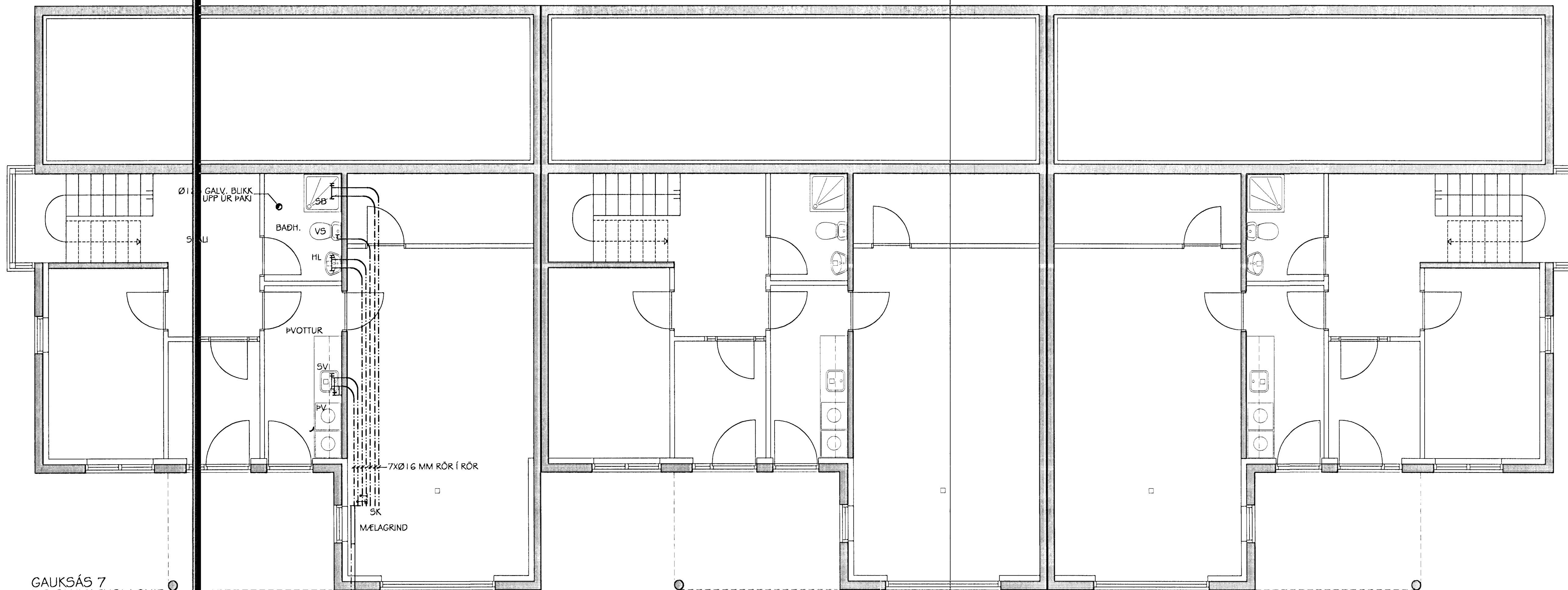
GAUKSÁS 7 NEYSLUVATNS- OG HEIÐLAGNIR FRÆRENNISLAGNIR OG LOFTRÆSING GRUNNMÝND EFRÍ HÆÐAR MKV. 1:50
