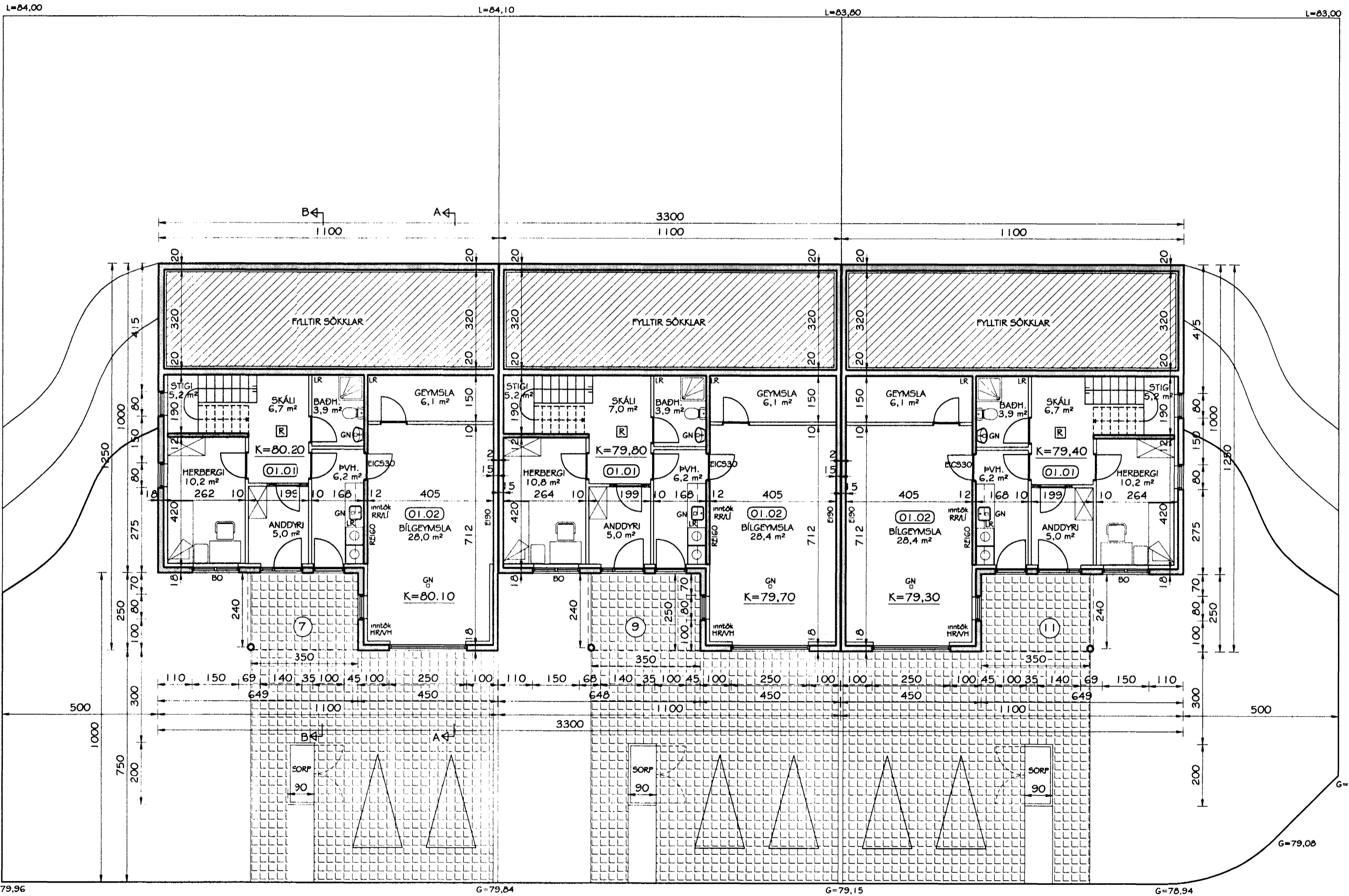
GRUNNMYND NEDRI HÆÐAR MKV. 1:100
