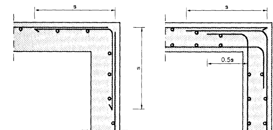
EINFÖLD BENDING
