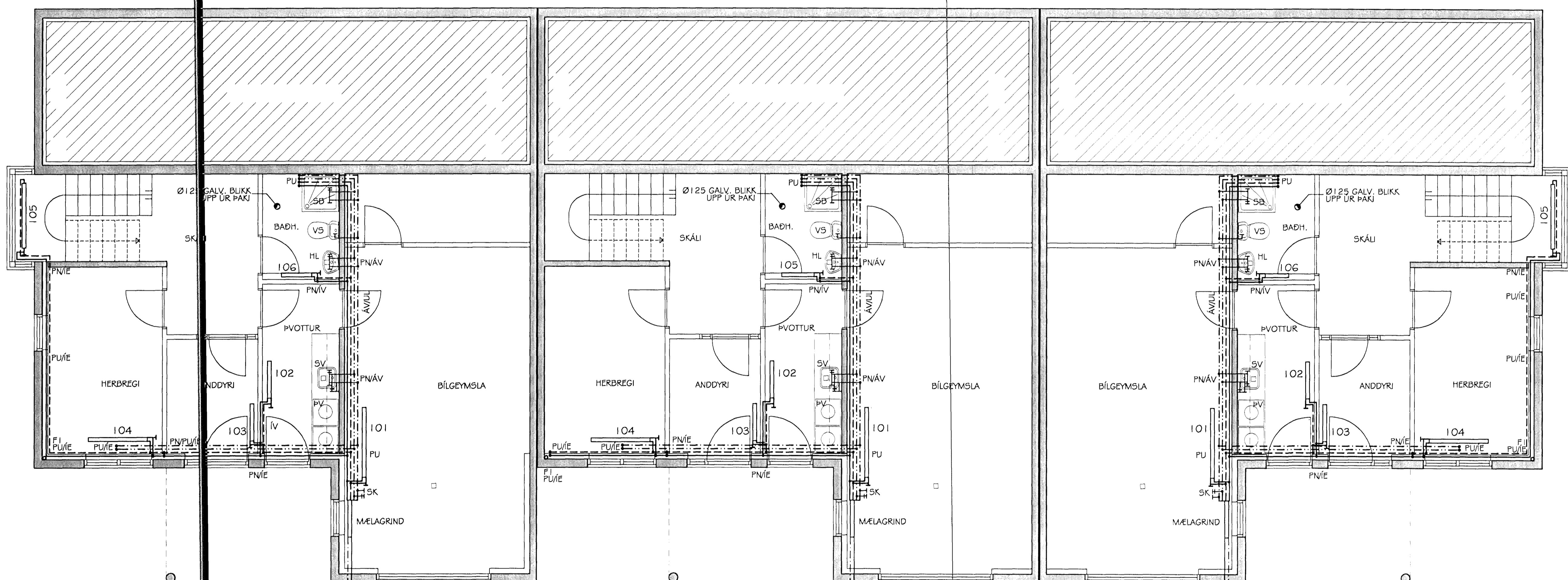
GAUKSÁS 7 NEYSLUVATNS- OG HITALAGNIR FRÆRENNISLAGNIR OG LOFTRÆSING GRUNNMÝND NEDRI HÆÐAR MKV. 1:50
