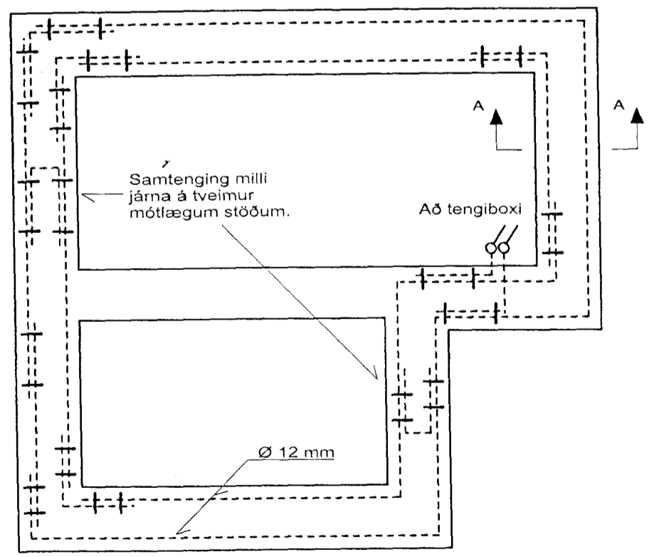
GRUNNMYND SÖKKULVEGGJA
