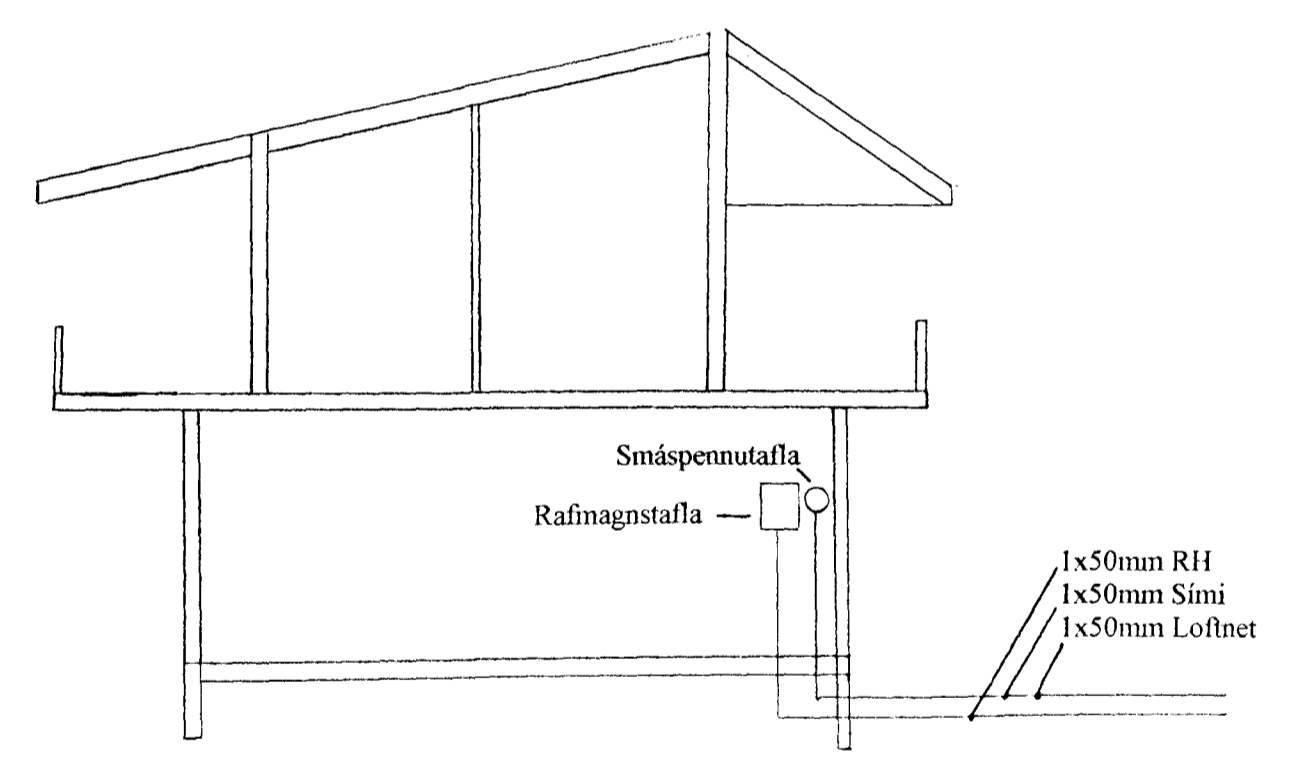
1:100 Inntakspípur 70 sm í jörð 3x50mm.
