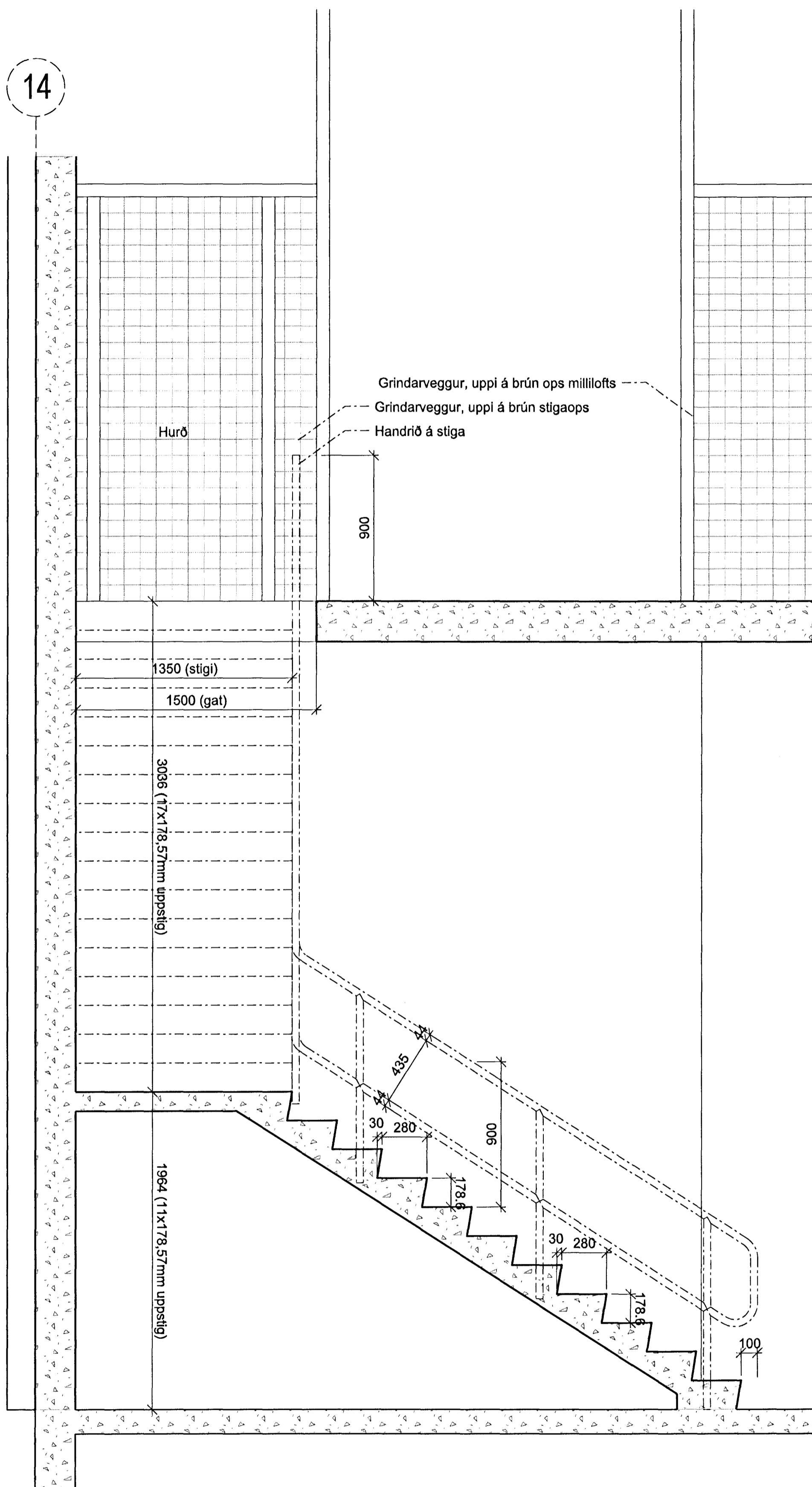
B-B 24-07 SNEIÐING 1:20 Stigi í nýjum lager
