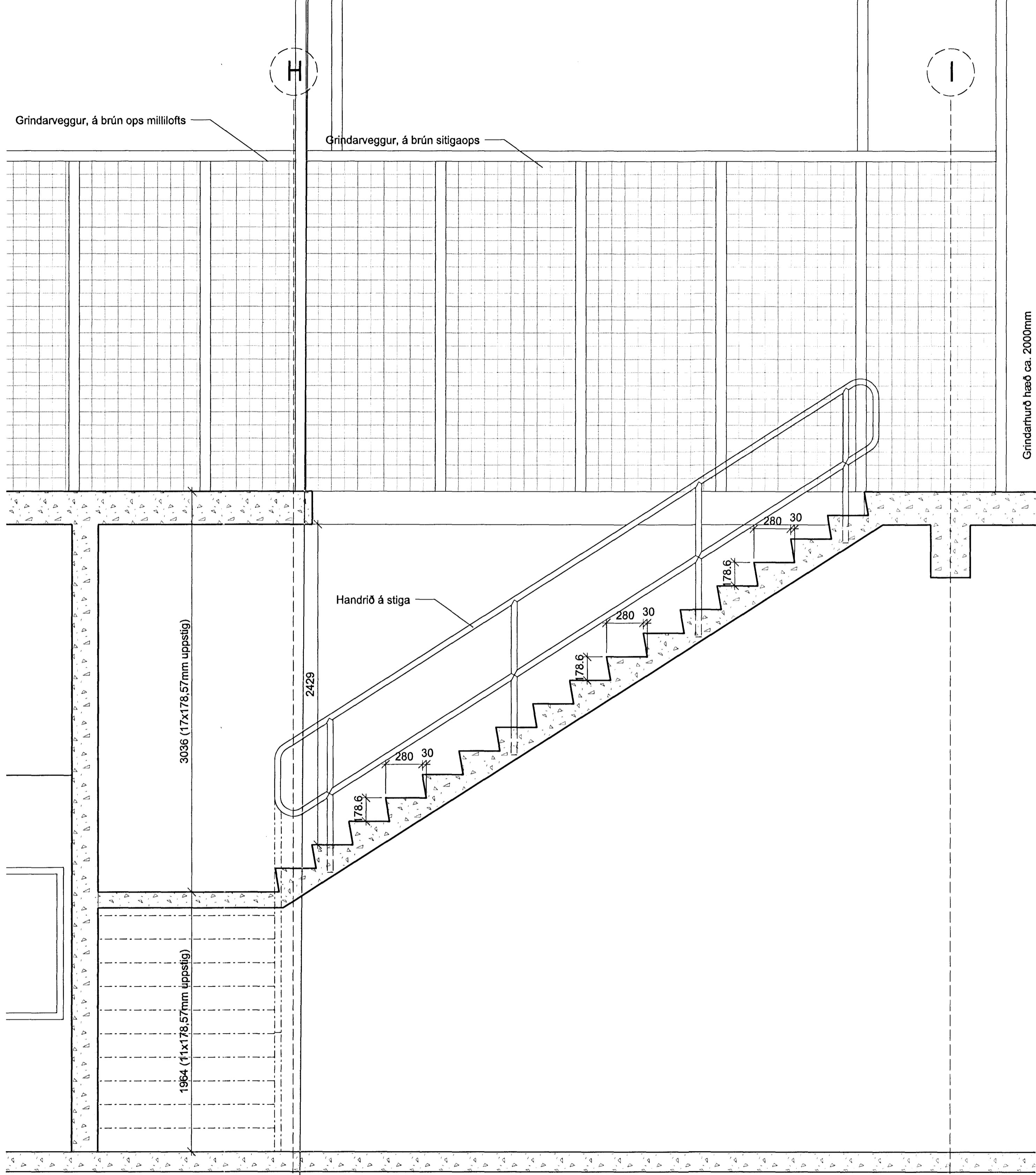
A-A 24-07 SNEIÐING 1:20 Stigi í nýjum lager
