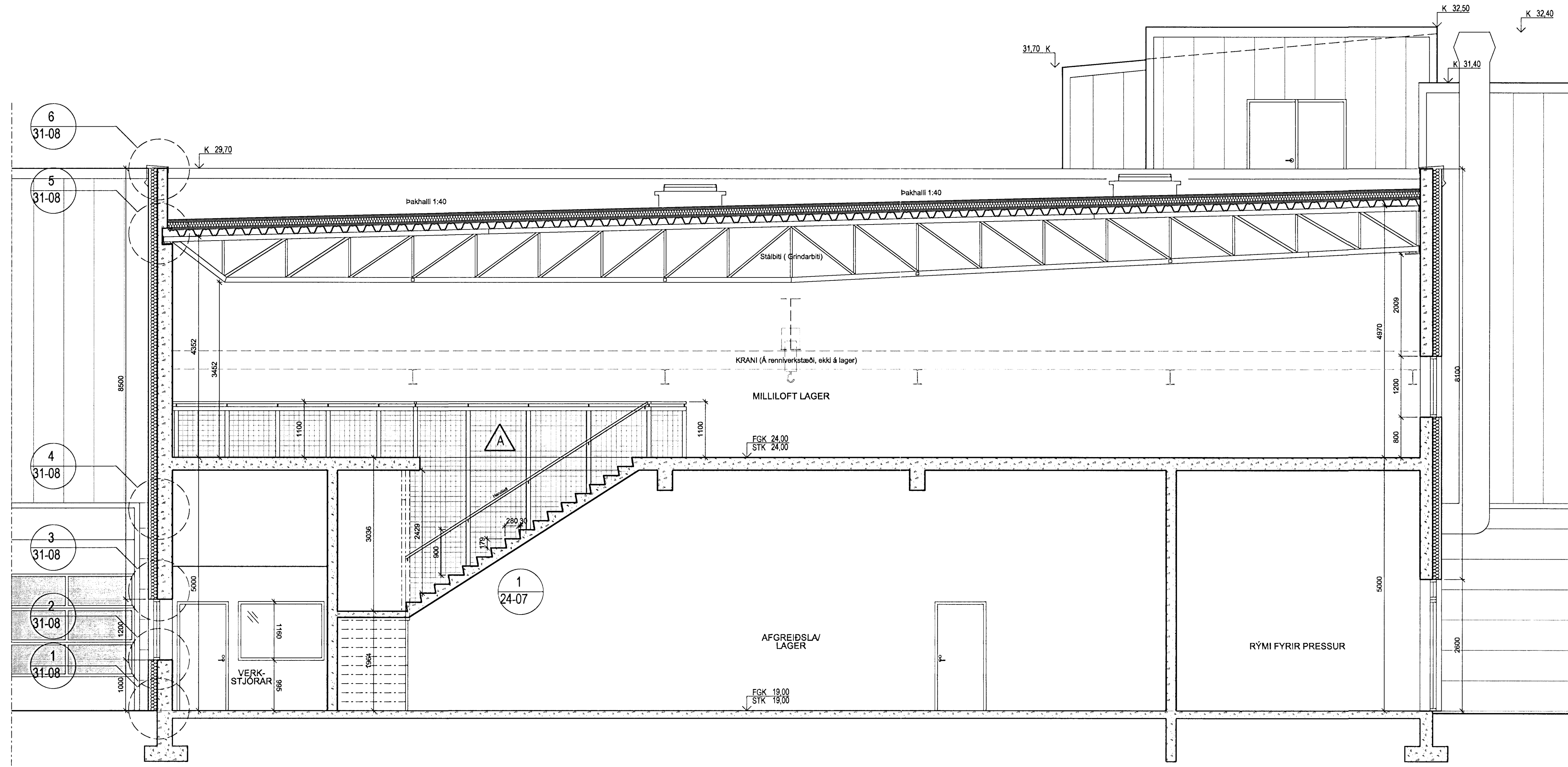
1 20-107 SNEIÐING 1:50 LAGER OG MILLILOFT YFIR LAGER
