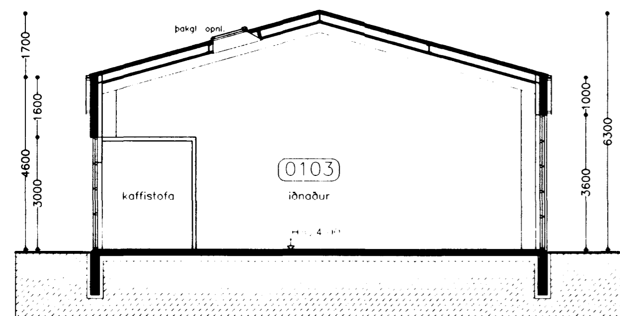
Þversnið B-B
