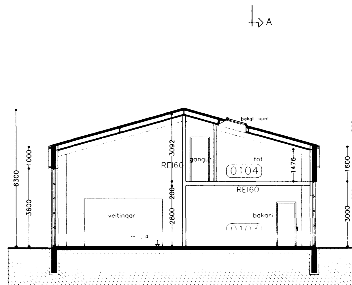
Þversnið A-A
