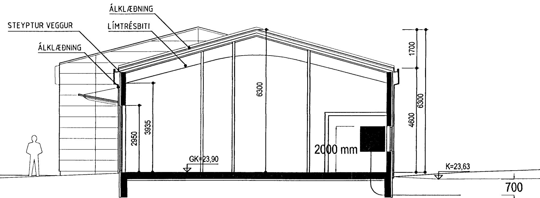
SNEIÐING A-A 1:100
