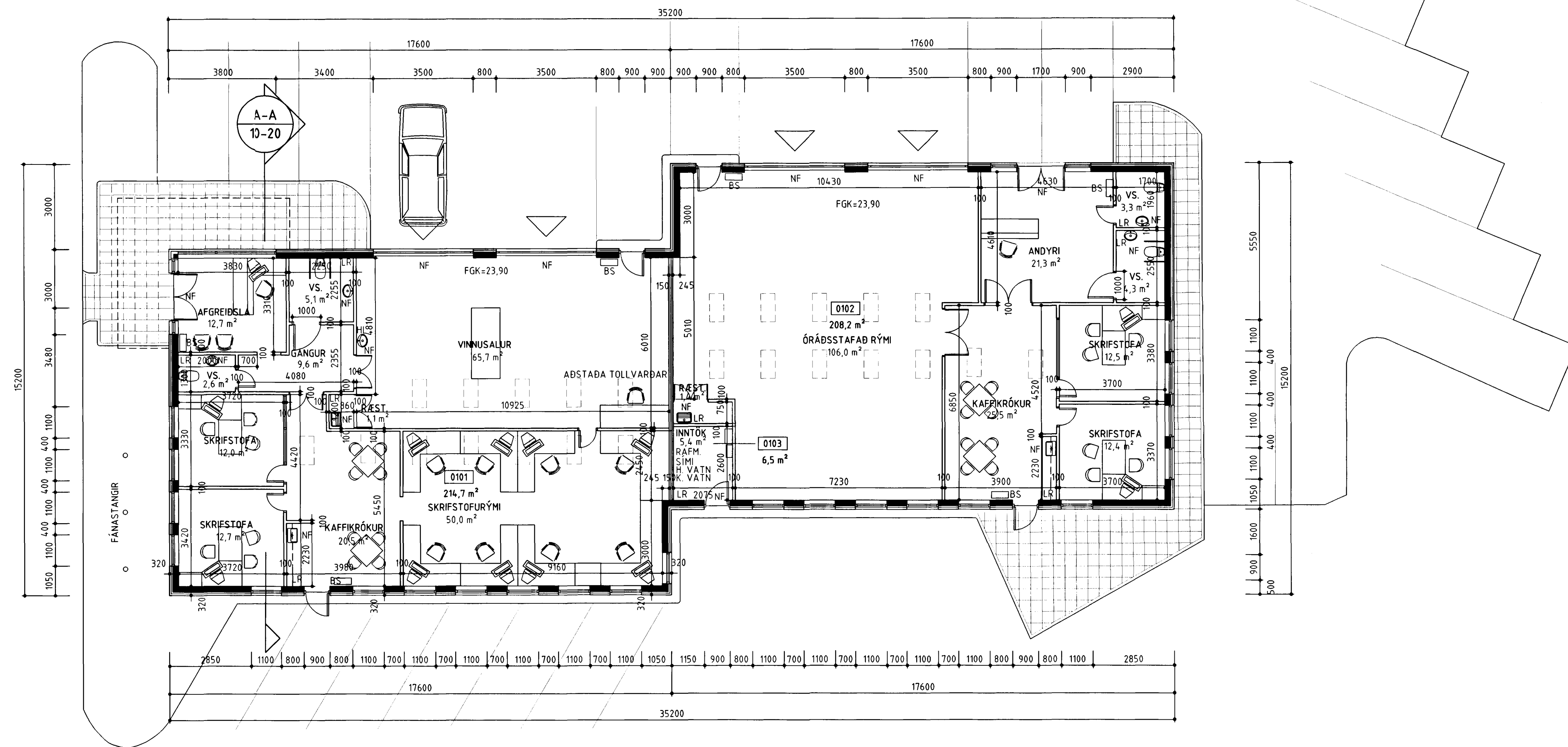
GRUNNMYND 1.HÆÐ 1:100
