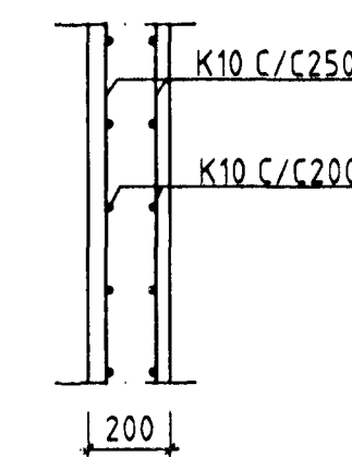
ALMENNT SNID Í V1 OG V2, M 1:20
