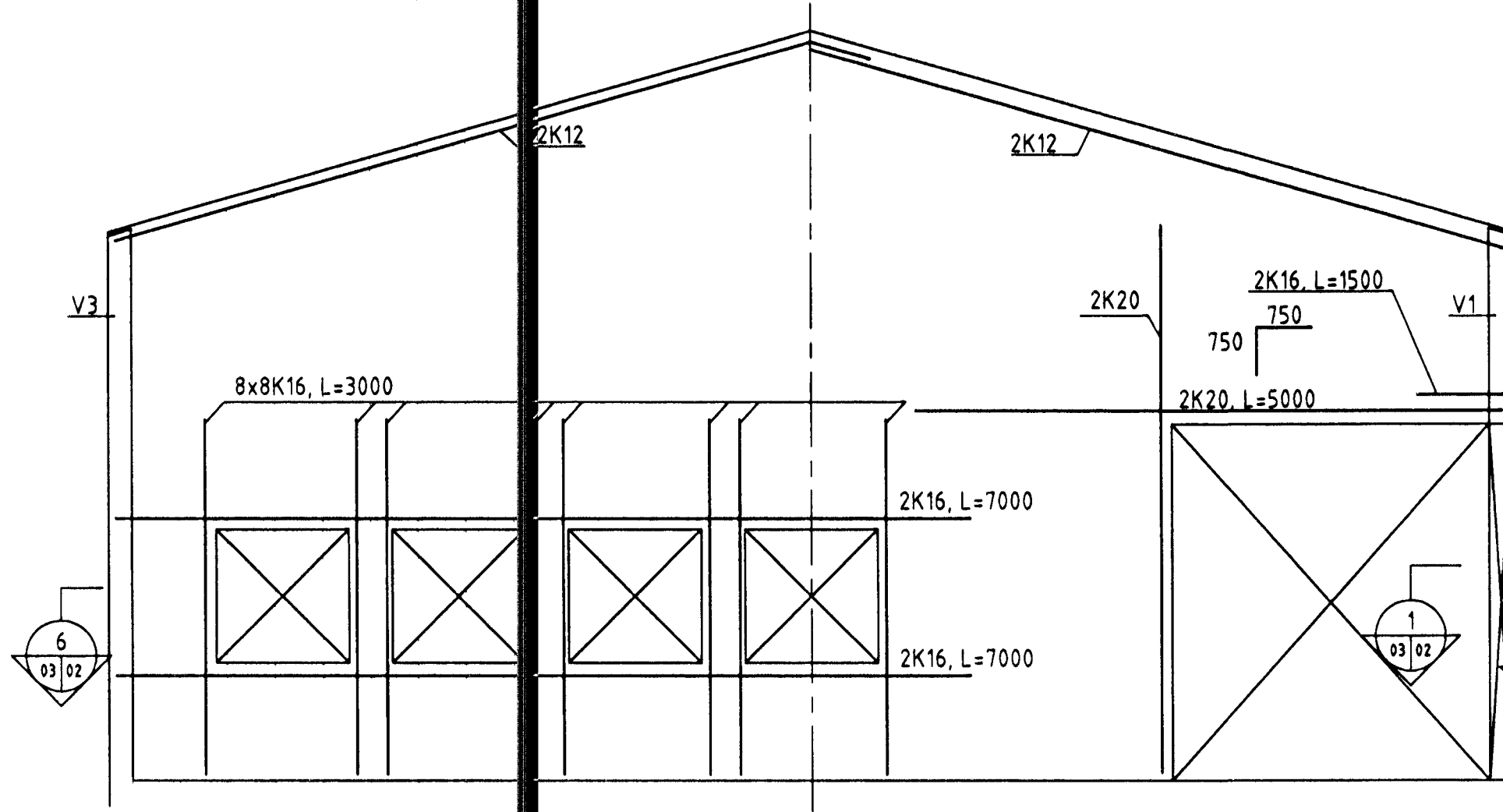
VEGGUR V3 (SÉÐ Á VEGGINN INNANFRÁ) M 1:50
