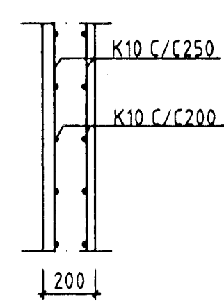
ALMENNT SNID Í V1 OG V2, M 1:20
