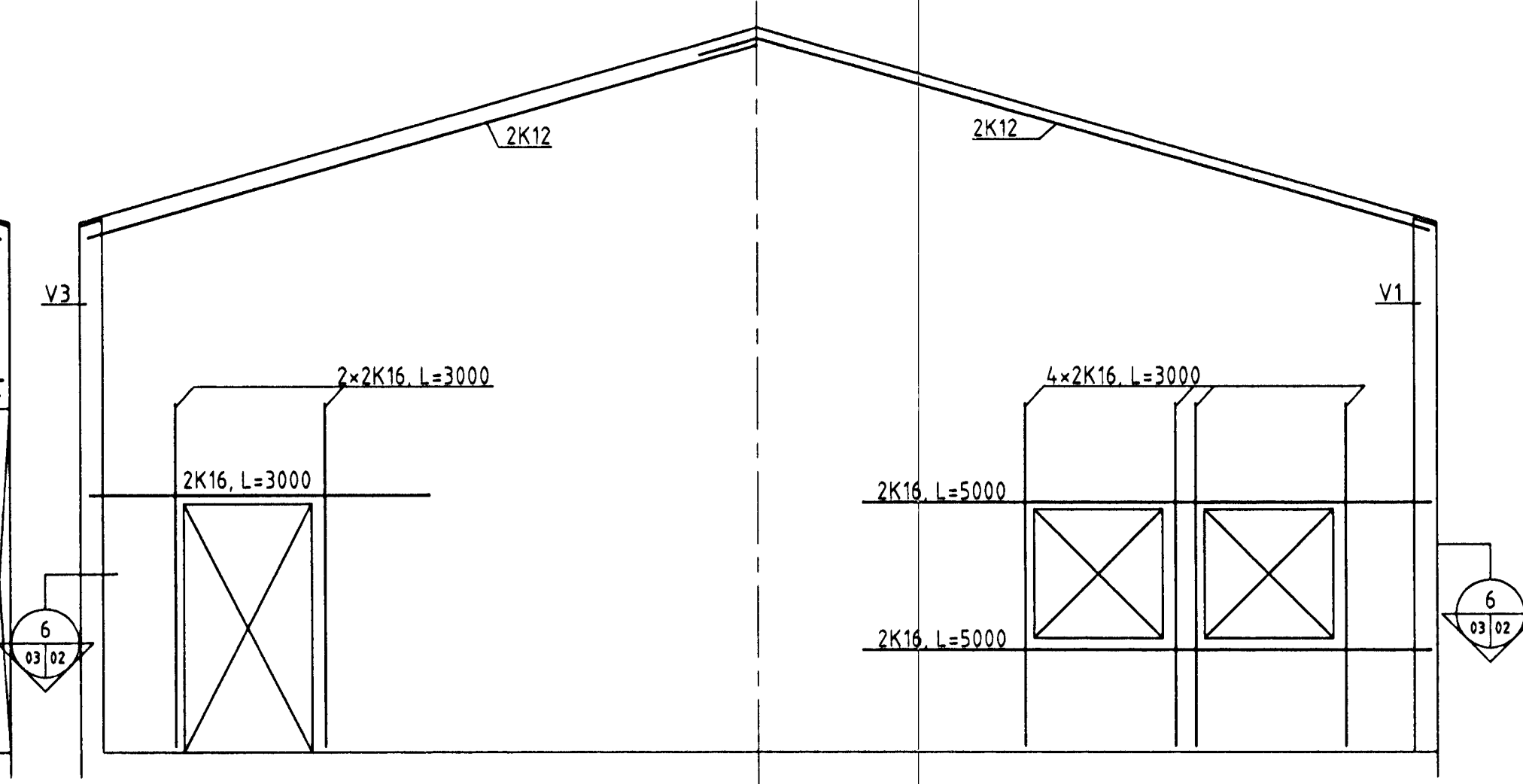
VEGGUR V4 (SÉÐ Á VEGGINN INNANFRÁ) M 1:50
