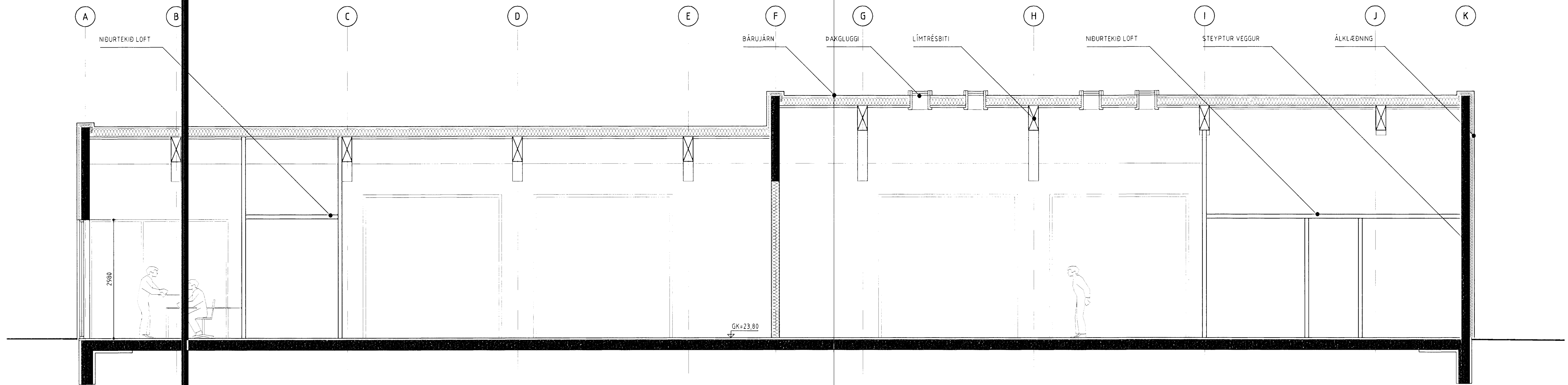
SNEIDING A-A 1:50
