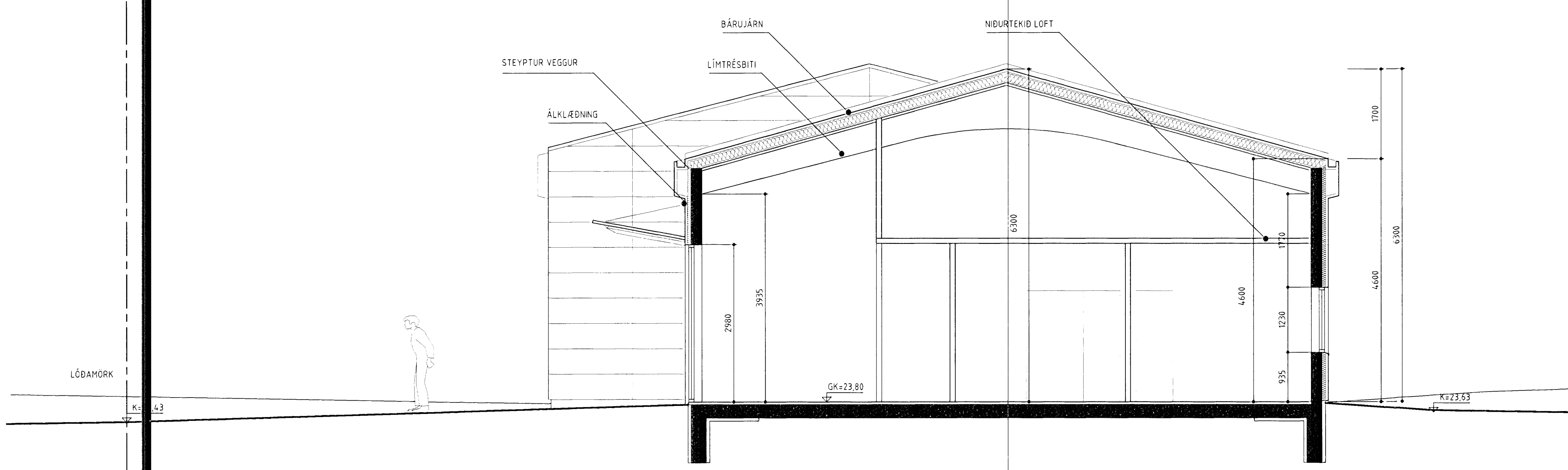
SNEIDING B-B 1:50
