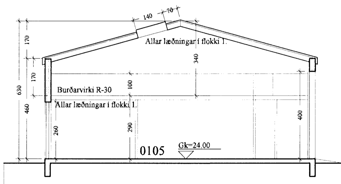
SNEIÐING a-a 1:100
