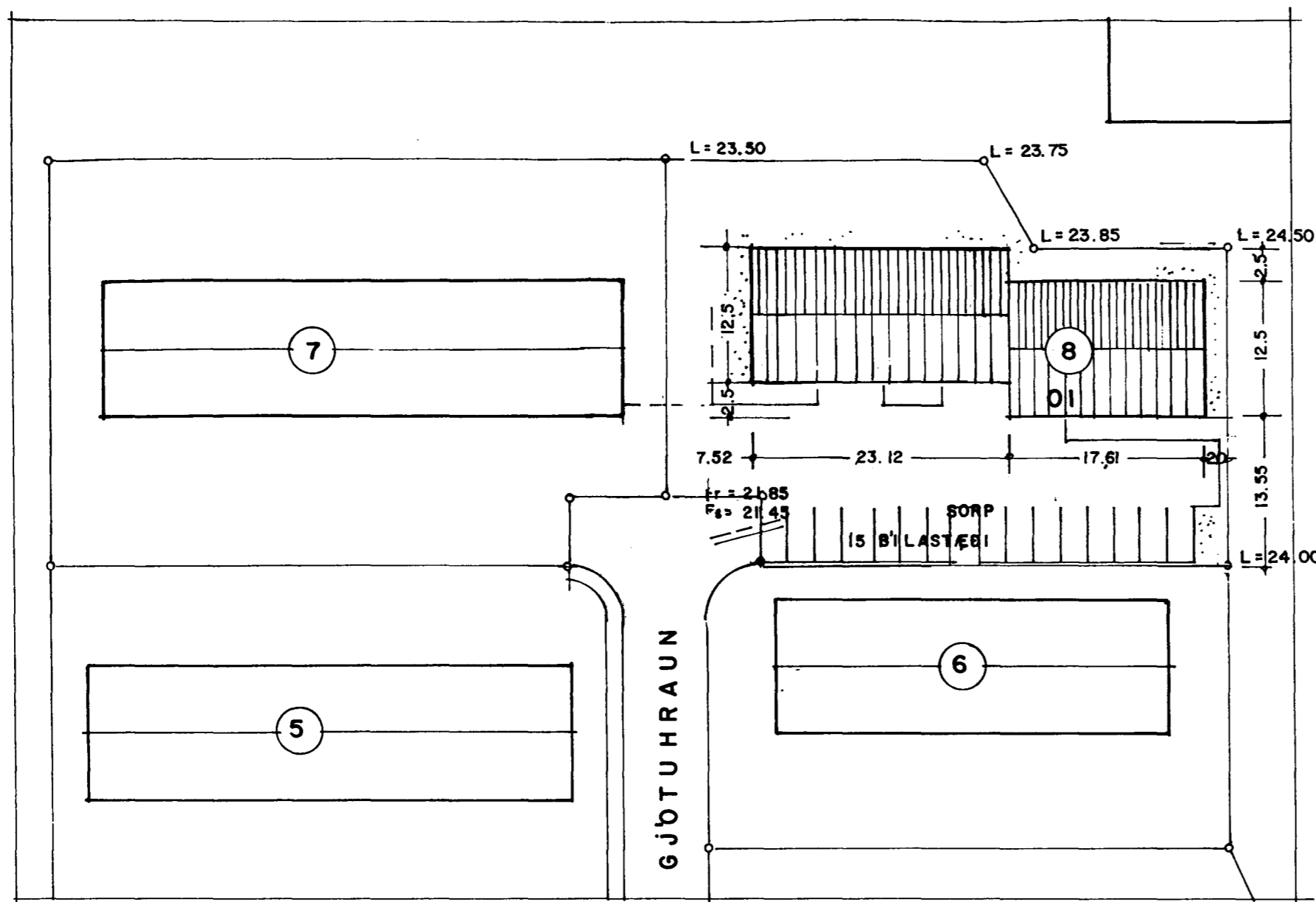
AFSTÖÐUMYND 1 : 500
