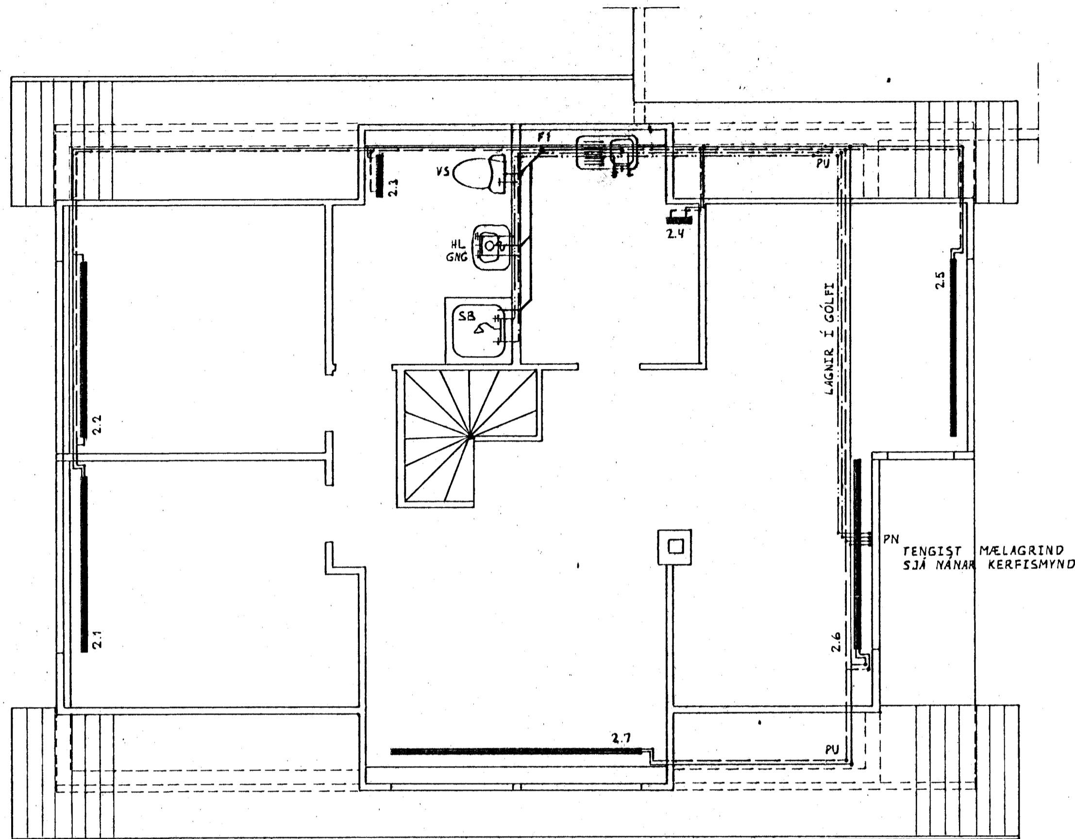
GRUNNMYND 1:50
