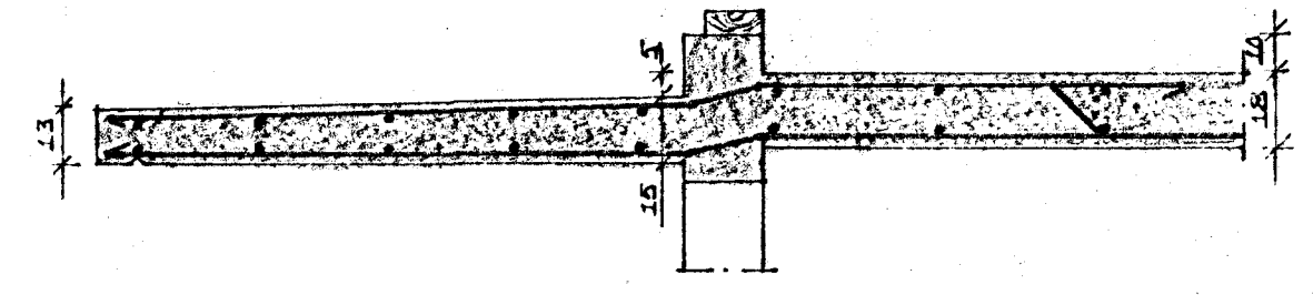
SNID A-A 1:20
