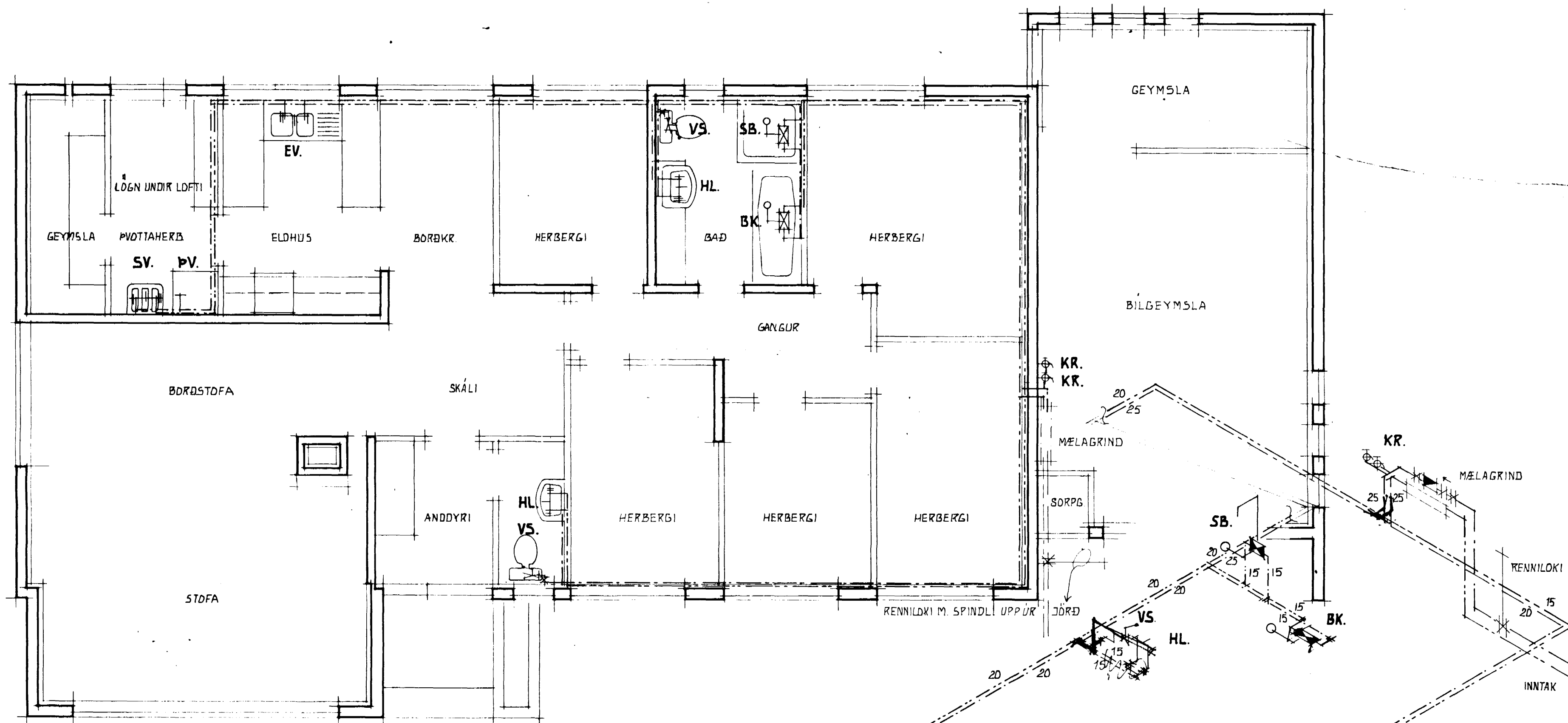
GRUNNMYND MK. 1:50
