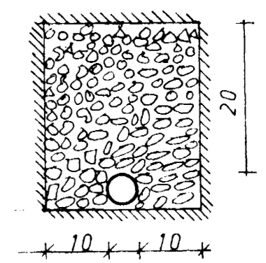
JARÐVATNSLÖGN ÞVERSNIÐ 1:10
