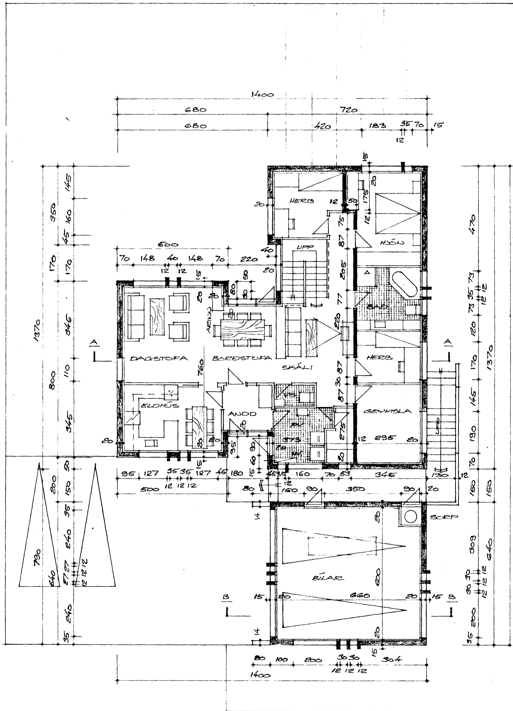
GRUNDMYND HÆÐAR, M=1:100
