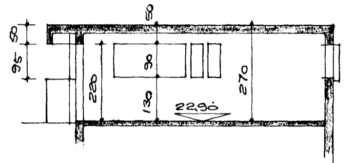
SKURÐUR B-B, M=1:100
