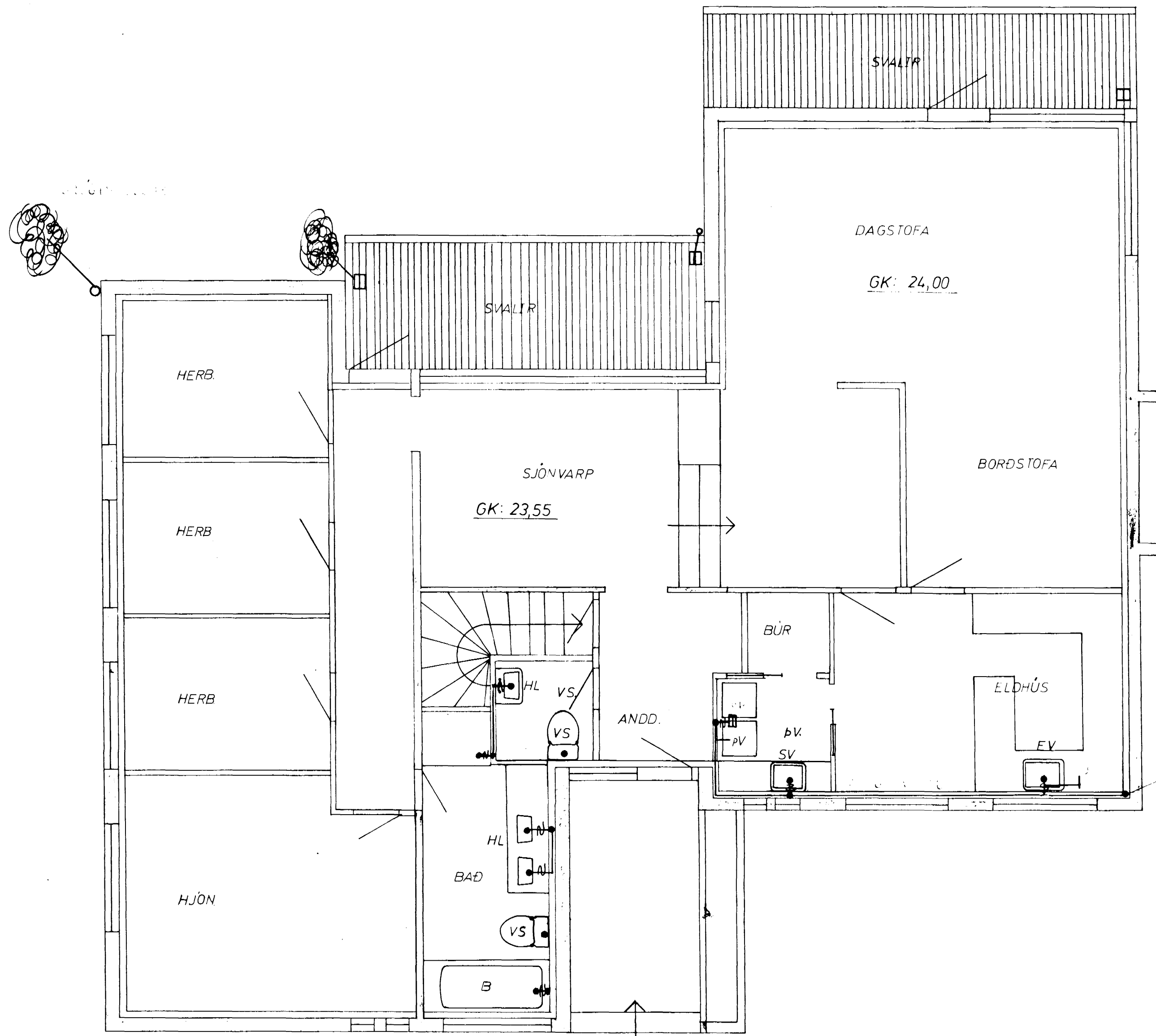
GRUNNMYND 1.HÆÐ 1:50
