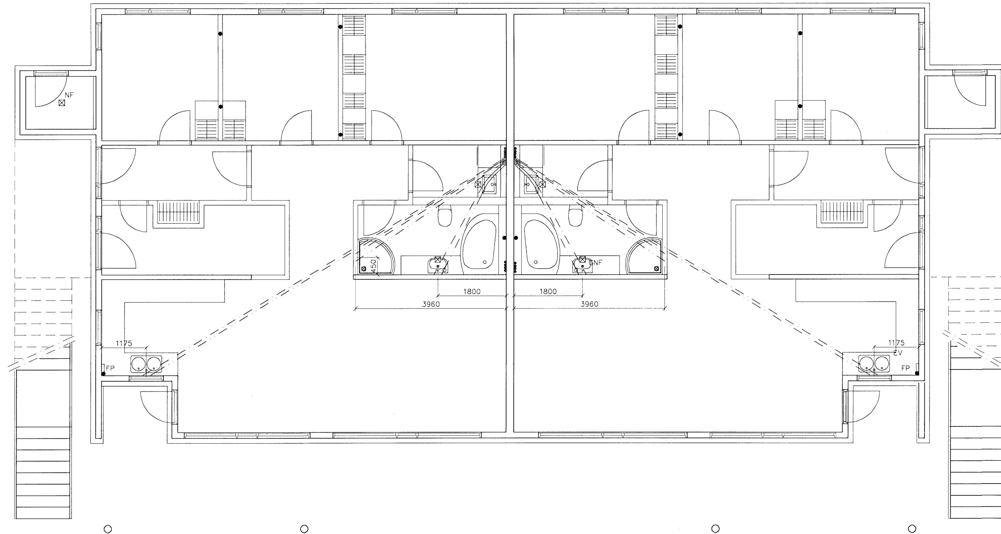
GRUNNMYND 1 HÆÐAR 1:50
