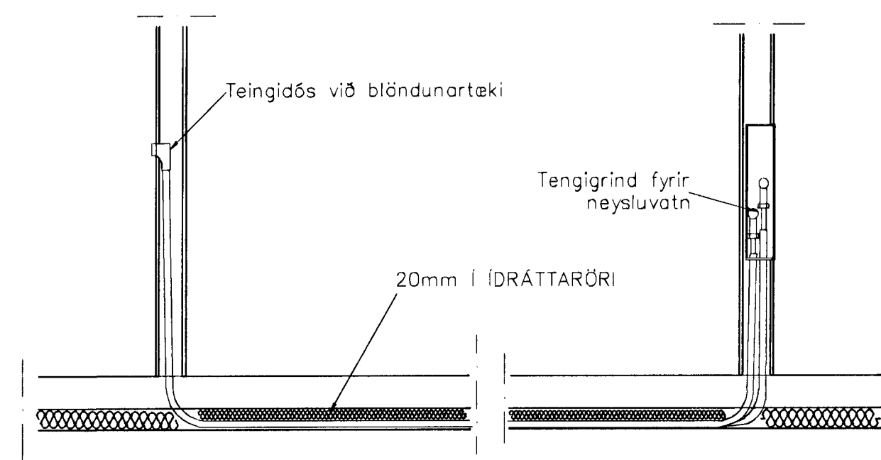
TENGING NEYSLUVATNSLAGNA 1:20
