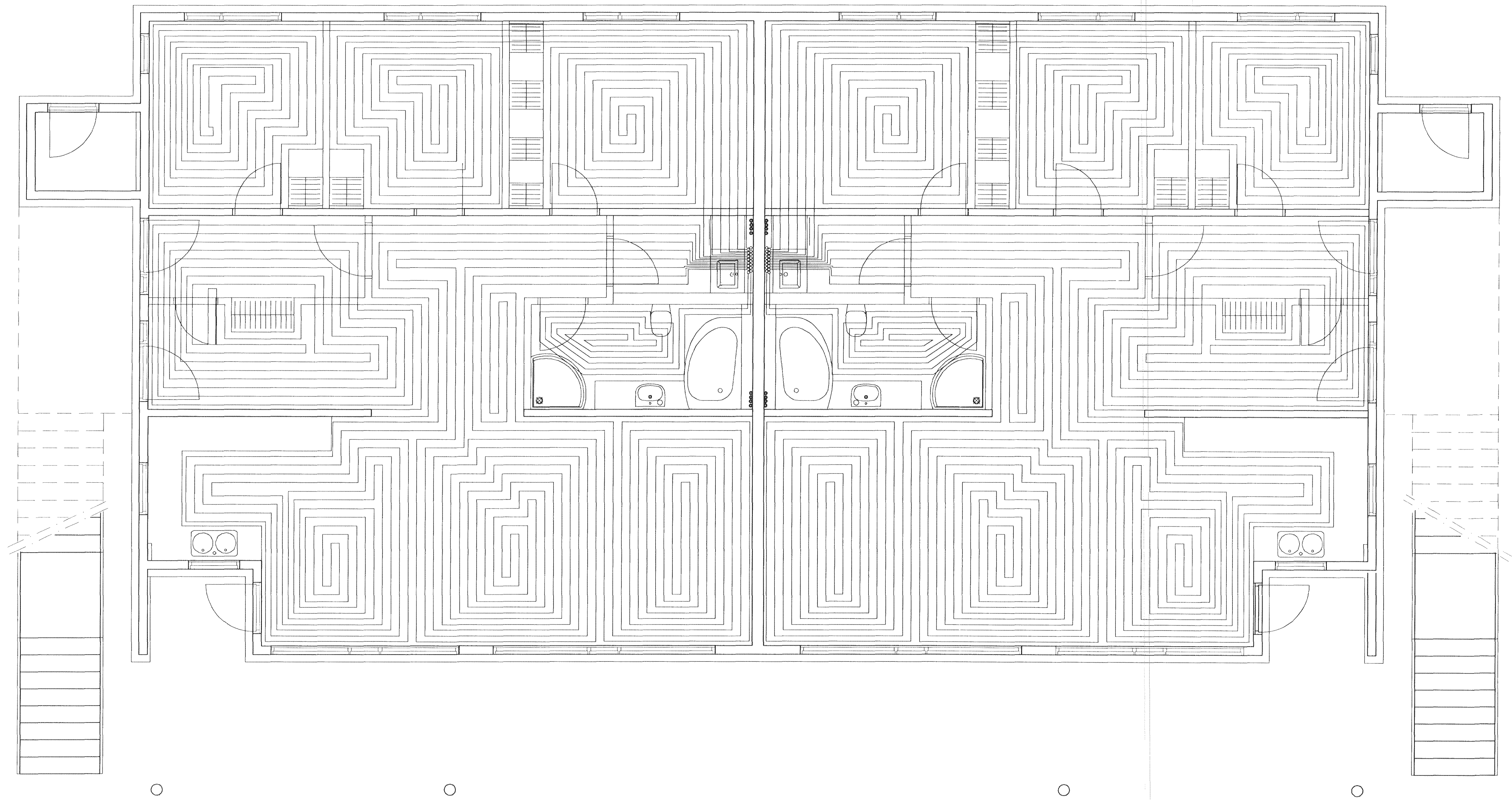
GRUNNMÝND 1 HÆÐAR 1:50
