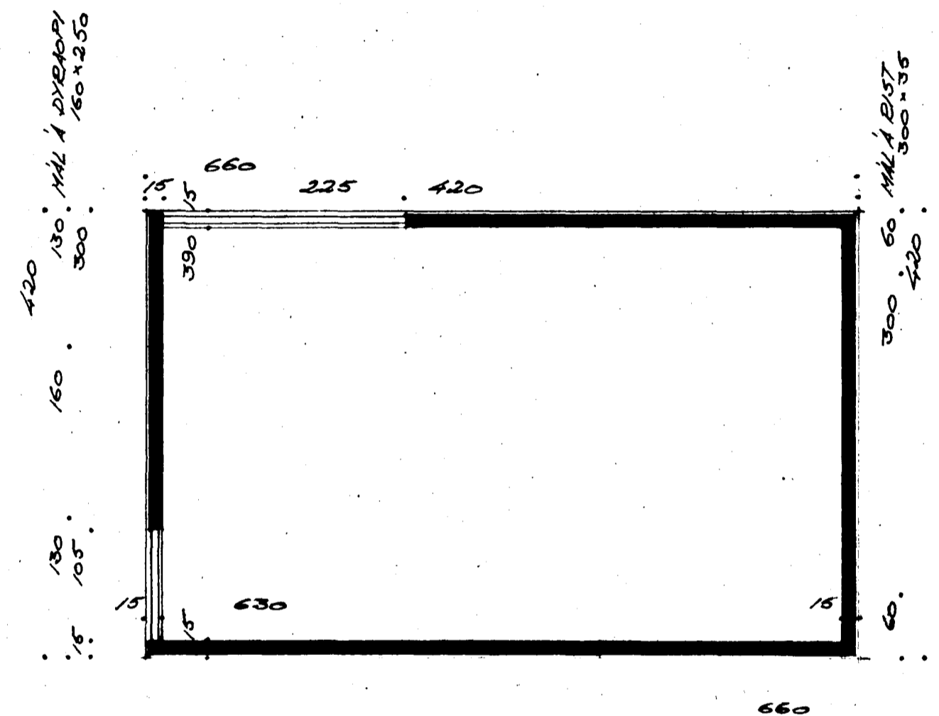
GRUNNMYND
