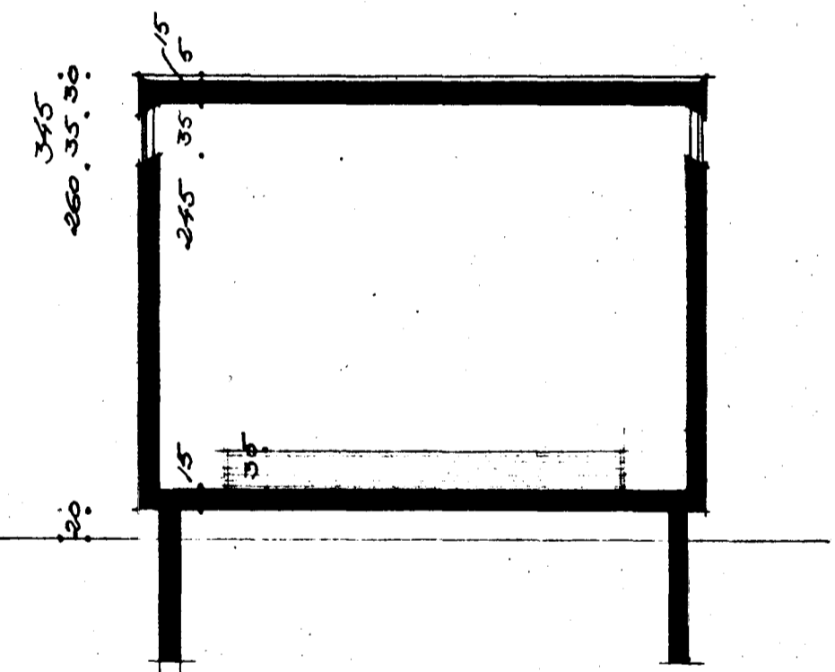
ÞVERSKURÐUR
