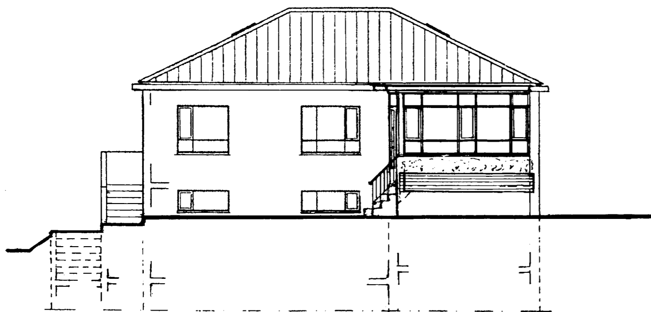
ÚTLIT MÓT SUÐ-VESTRI
