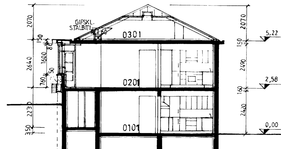
SNEIÐING B-B
