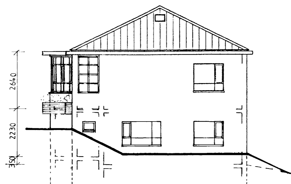
ÚTLIT MÓT SUÐ-AUSTRI
