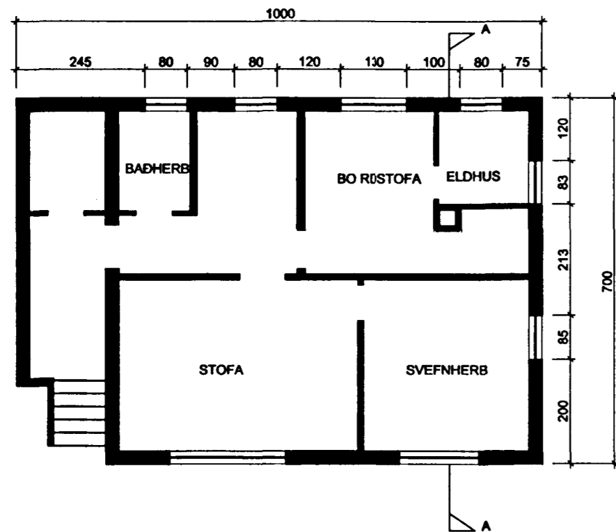
GRUNNMYND KJALLARA 1:100
