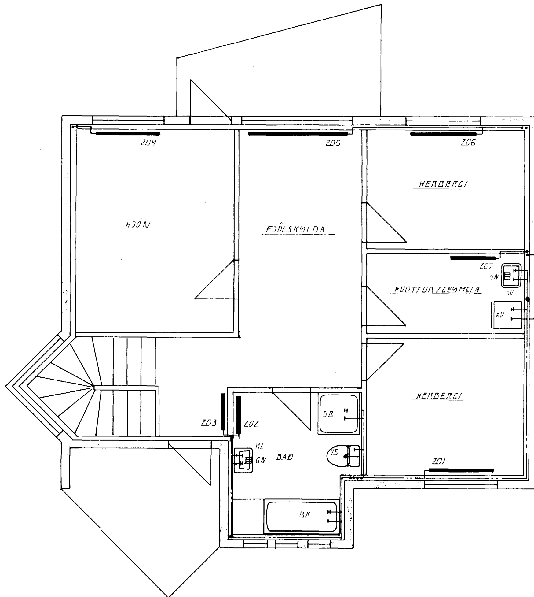
GRUNNMÝND . 2. HÆÐ . 1:50
