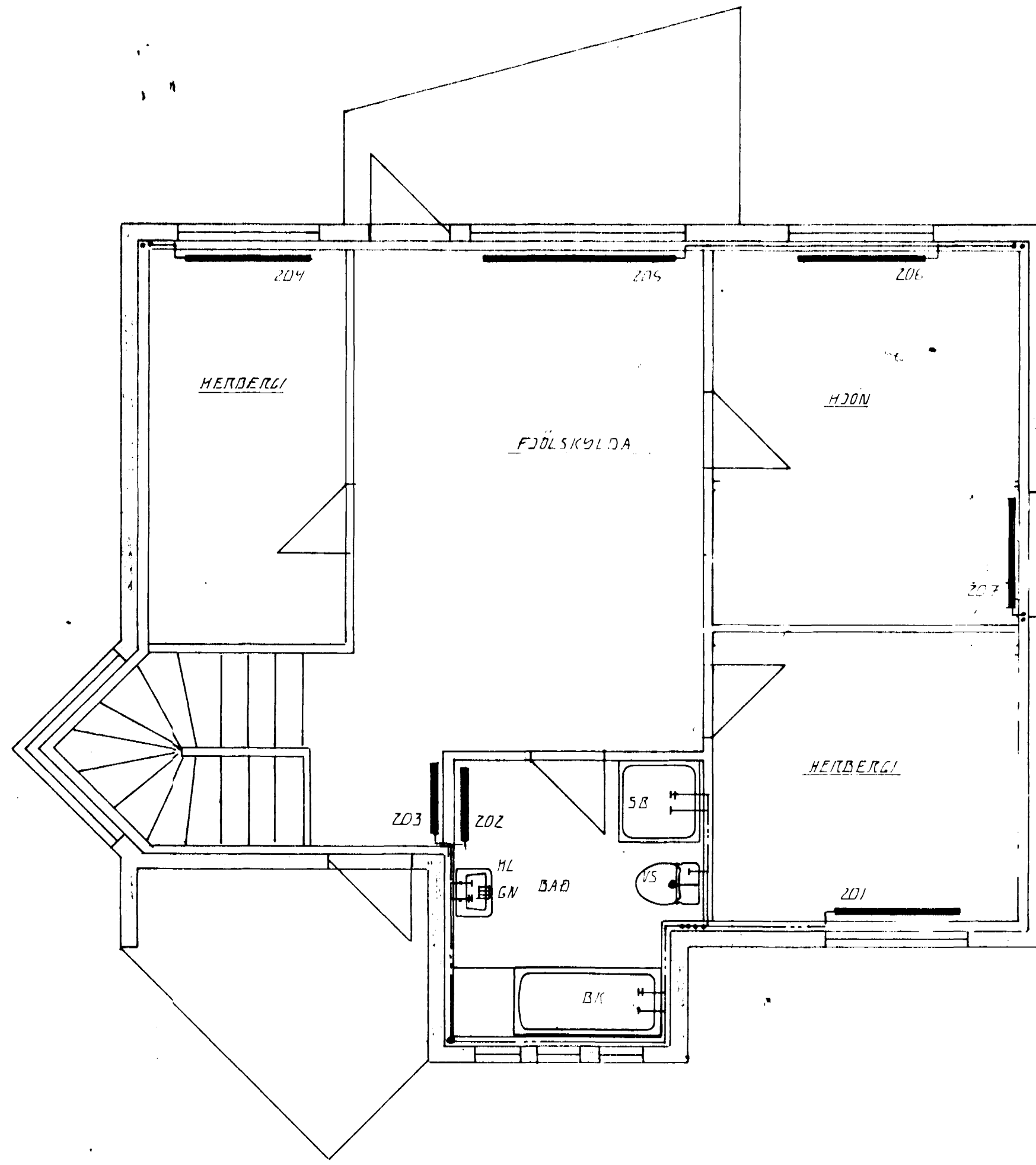
GRUNNMÝND, 2. HÆÐ, 1:50
